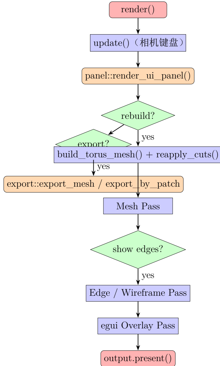
图 6: 渲染循环流程
