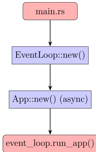
图 1: 程序入口流程
