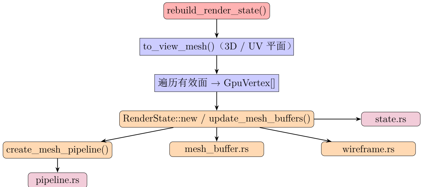
图 5: 渲染状态构建流程
