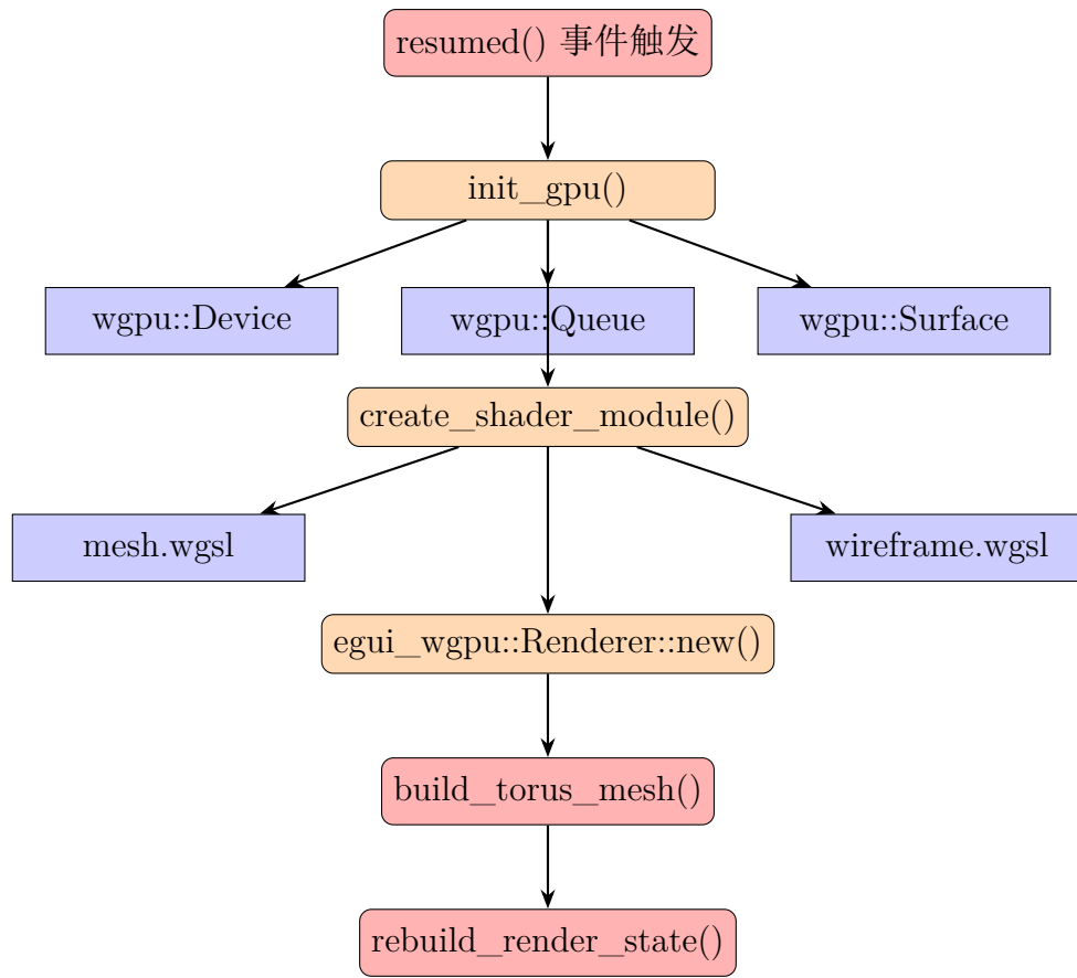
图 2: App 初始化流程 (App::new 为 async; GPU/着色器/egui 在 resumed 中创建)
