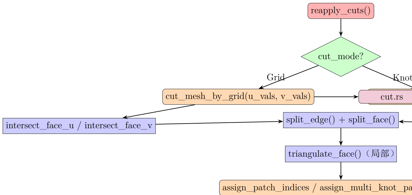
图 4: 切割与补片分配流程 (Grid / Knot 两种模式)
