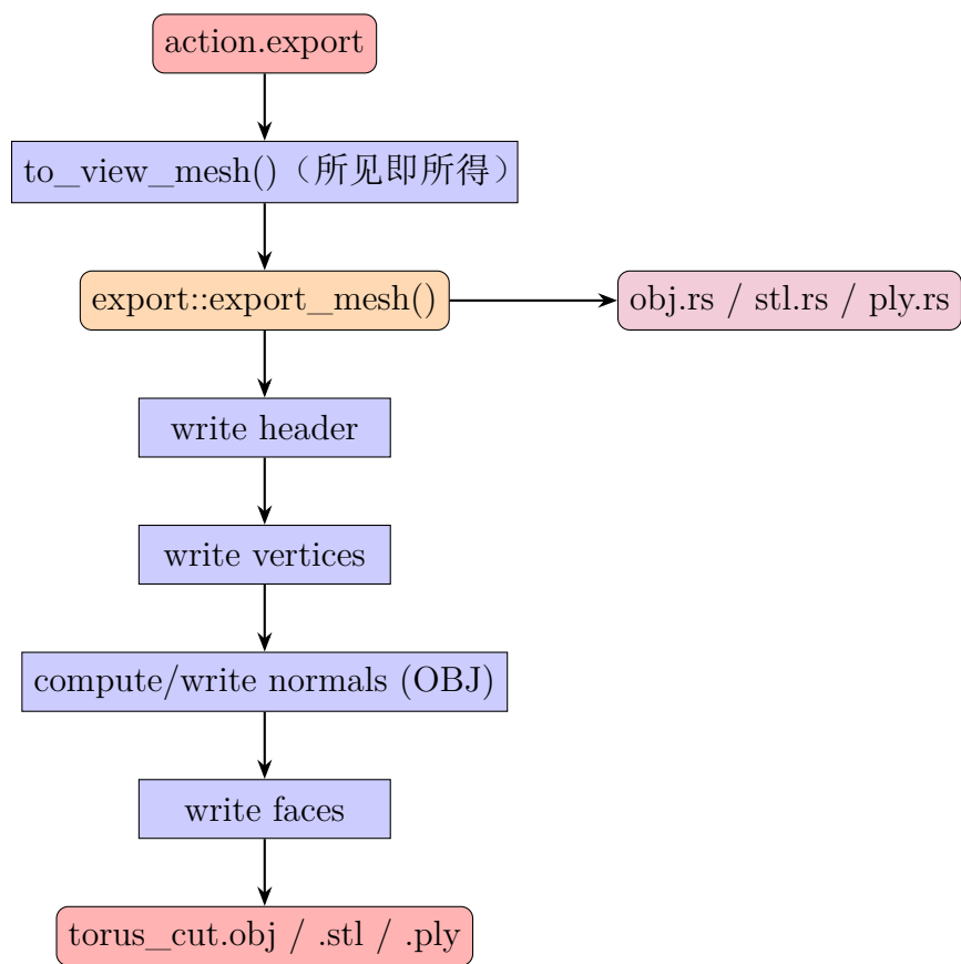
图 8: 导出流程 (OBJ / STL / PLY, 按 patch 时每片一个文件)
