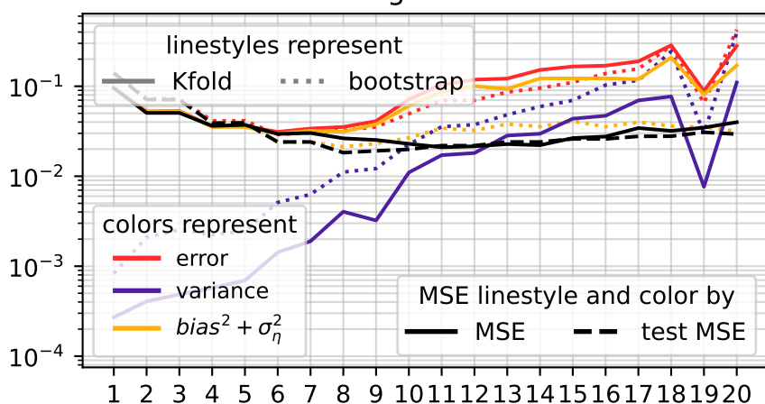
Lasso k = 5
