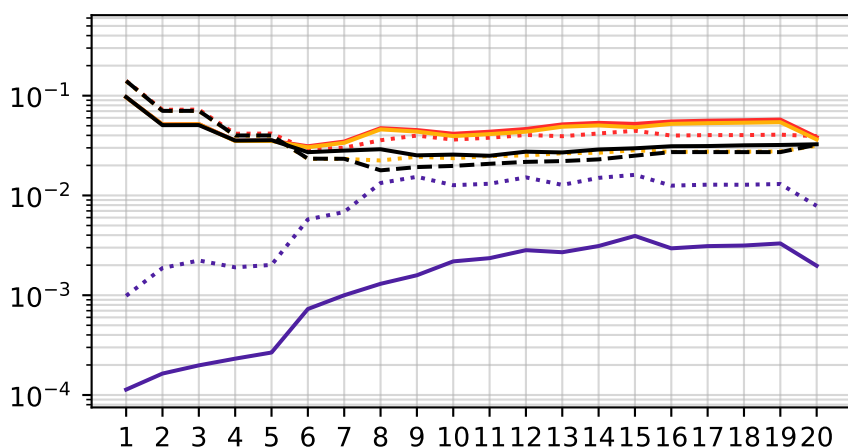
Lasso k = 10
