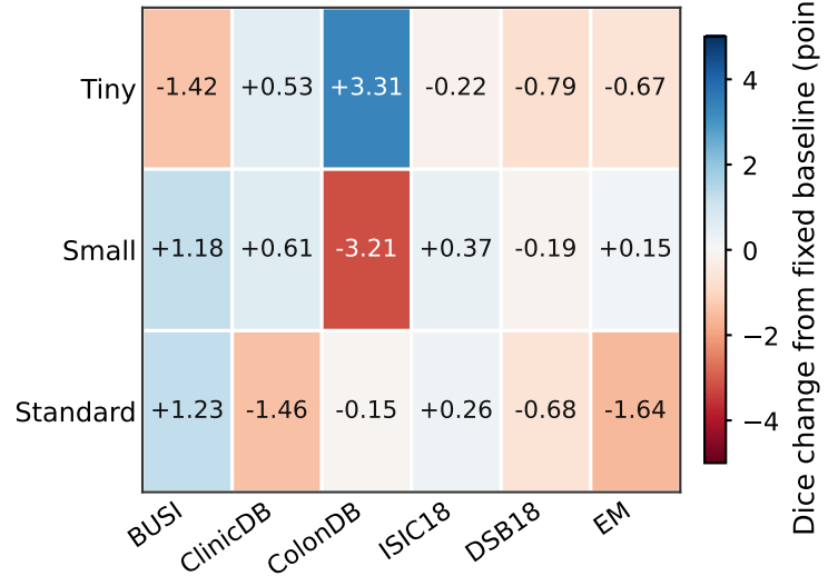
Sparse top-1
