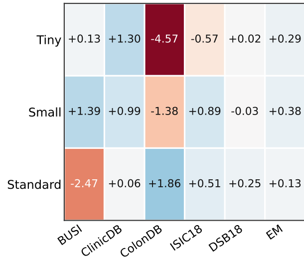
Static {3, 5}
