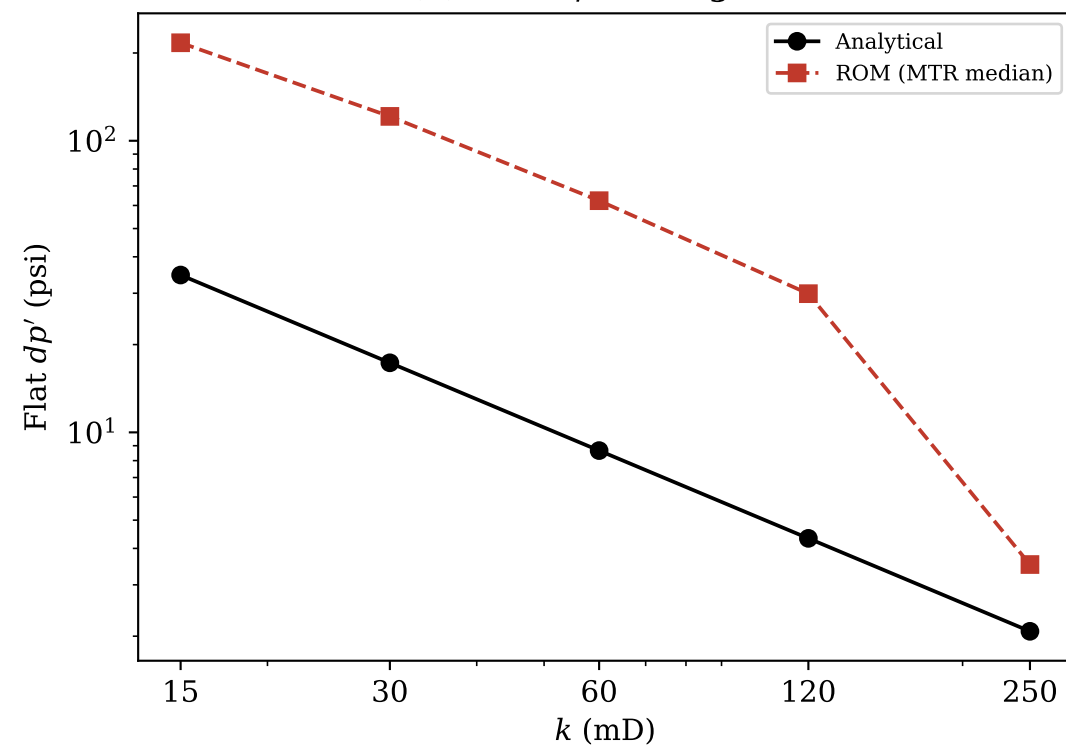
(D) Flat dp' scaling vs k
