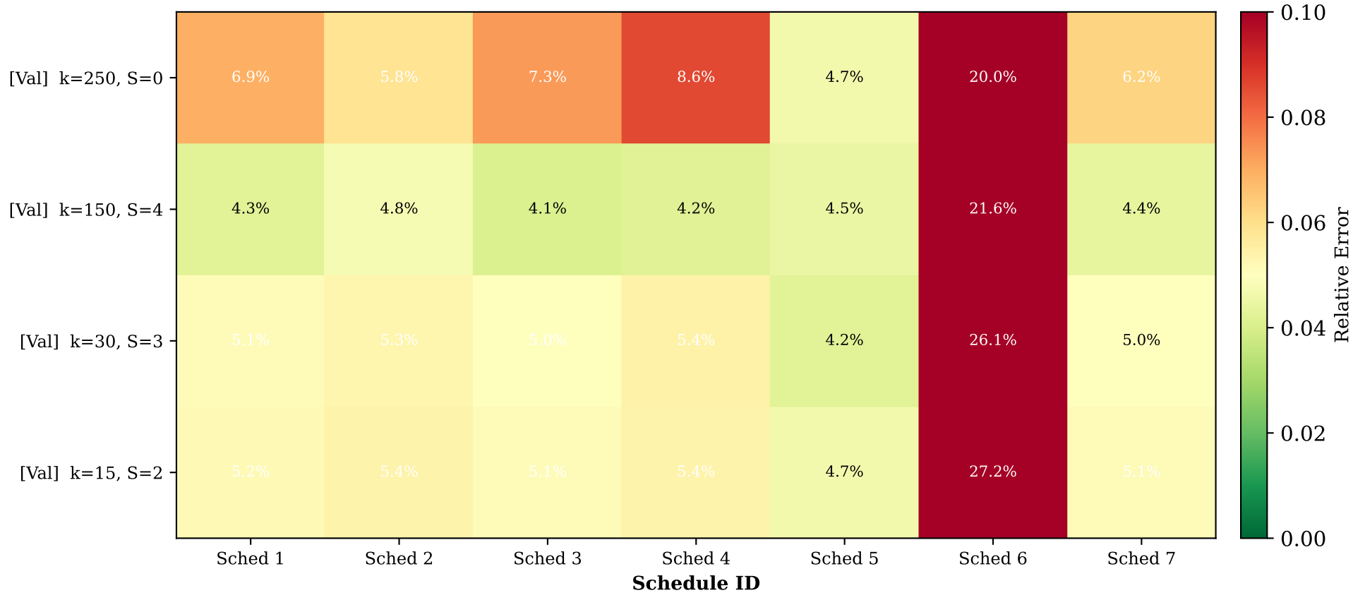
Relative Output Error: \|\Delta p_{\text{ROM}} - \Delta p_{\text{MRST}}\| / \|\Delta p_{\text{MRST}}\|
