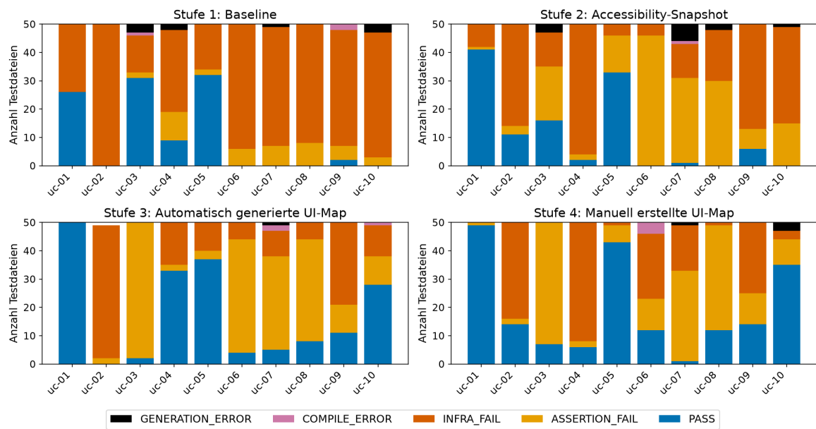
Abbildung 7: Ausführungskategorien je Use Case, Stufen 1 bis 4 (Phase 1)
