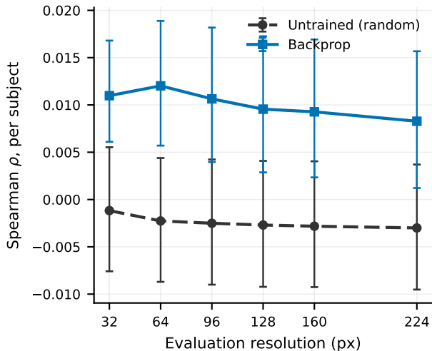
LOC (Conv3)
