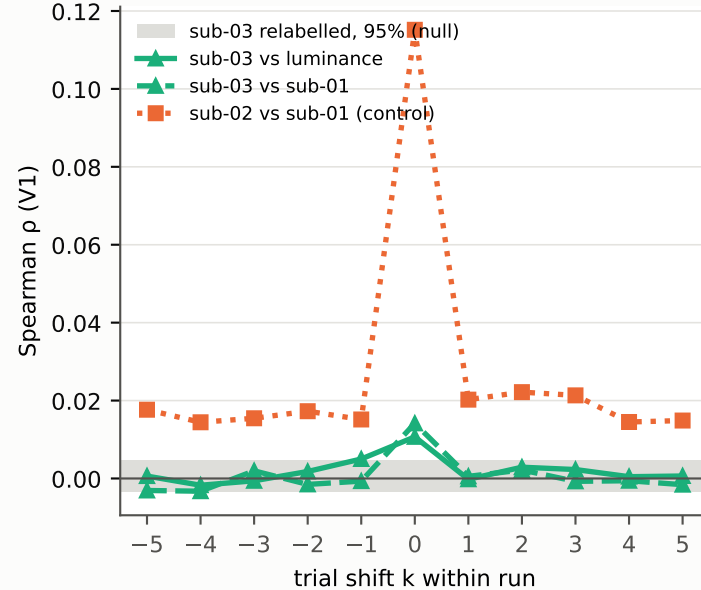
C Shift test, V1
