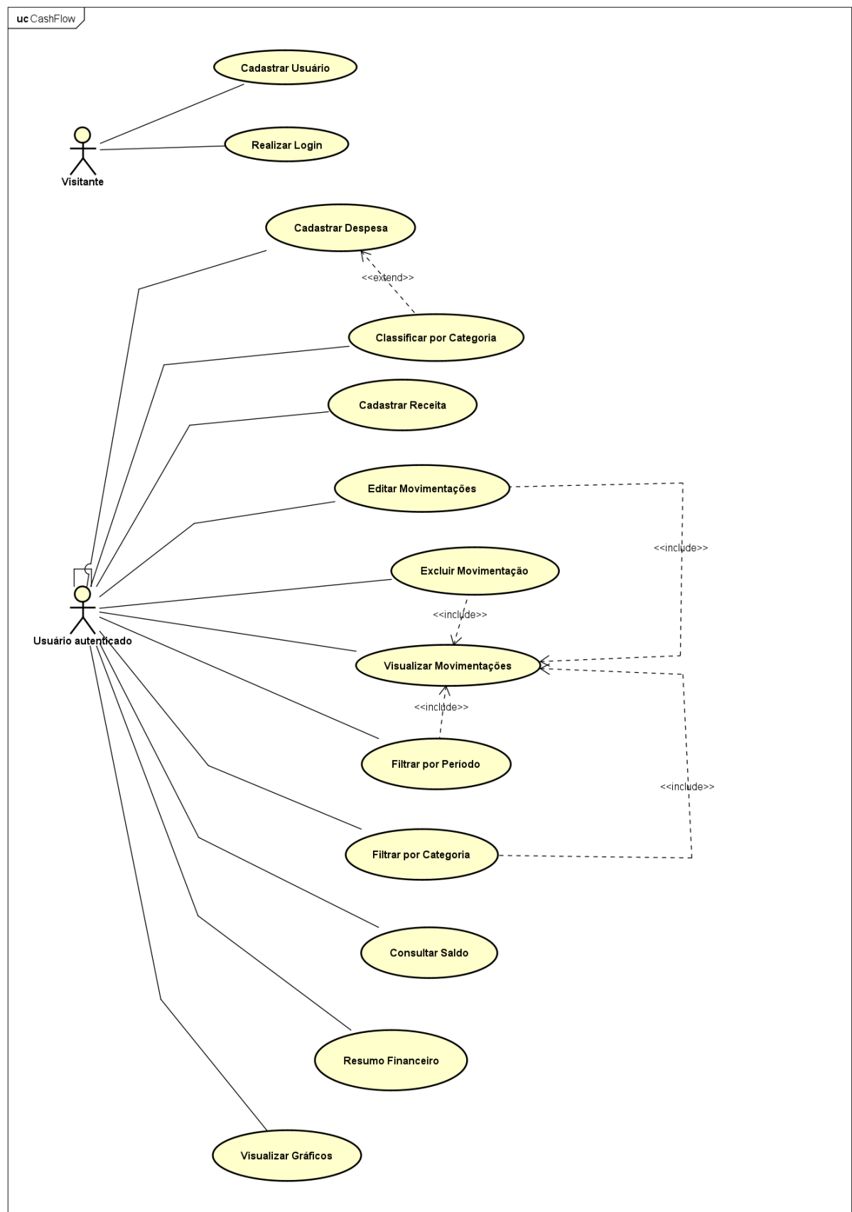
Figura 1: Diagrama de Casos de Uso do CashFlow
