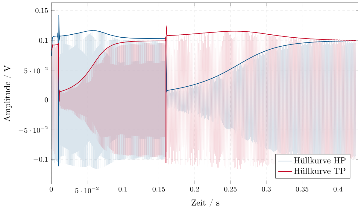
Abbildung 4.4: Amplituden-Einschwingverhalten des Biquads für Hoch- und Tiefpass
