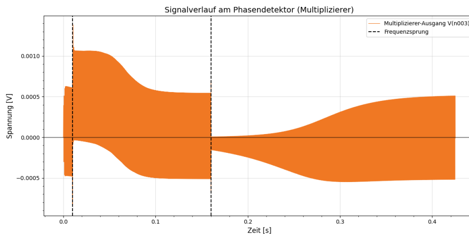
Abbildung 4.3: Signalverlauf am Multiplizierer im Phasendetektor
