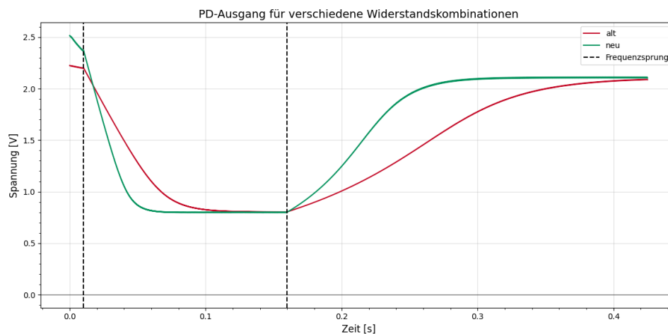
Abbildung 4.9: PD-Ausgang für verschiedene Widerstandskombinationen
