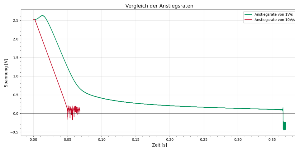
Abbildung 4.10: Vergleich der Steuerspannung bei unterschiedlichen Frequenzanstiegsraten
