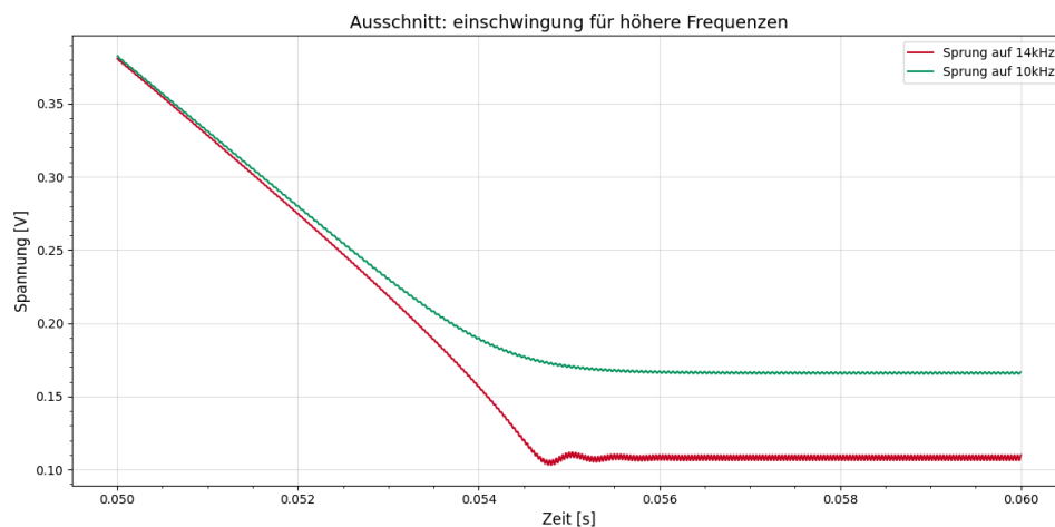
Abbildung 4.11: Einschwingverhalten der Steuerspannung für unterschiedliche Frequenzen
