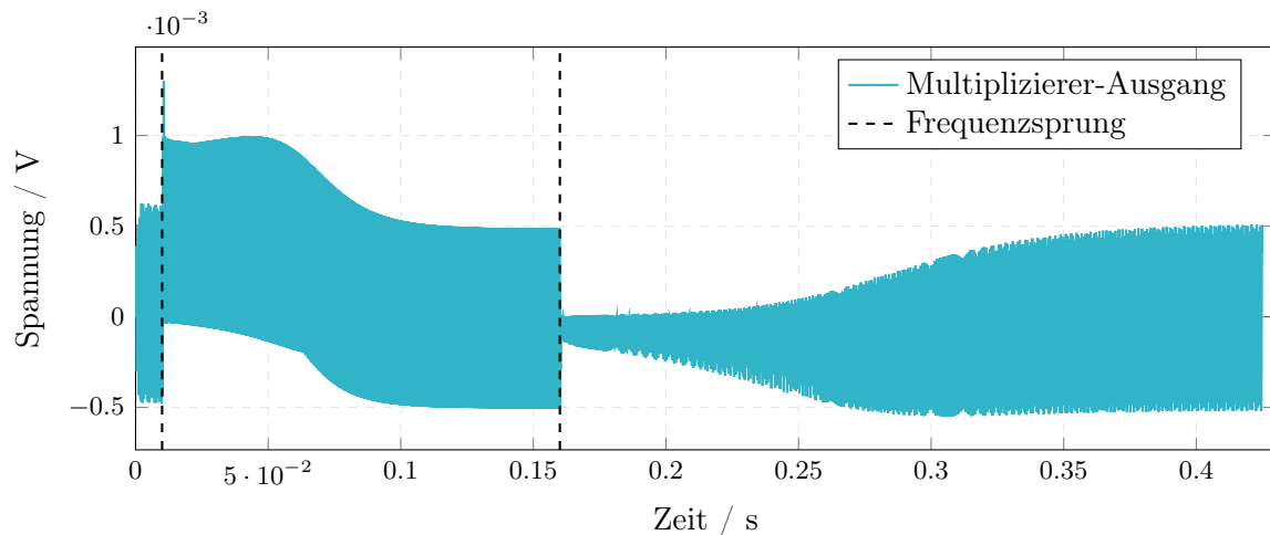
Abbildung 4.2: Signalverlauf am Multiplizierer im Phasendetektor
