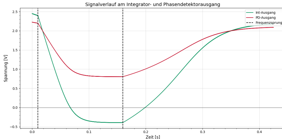
Abbildung 4.8: Spannungsvergleich am Integrator- und Phasendetektorausgang
