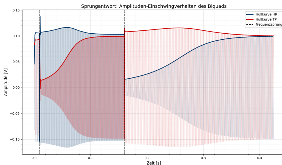
Abbildung 4.5: Amplituden-Einschwingverhalten des Biquads für Hoch- und Tiefpass
