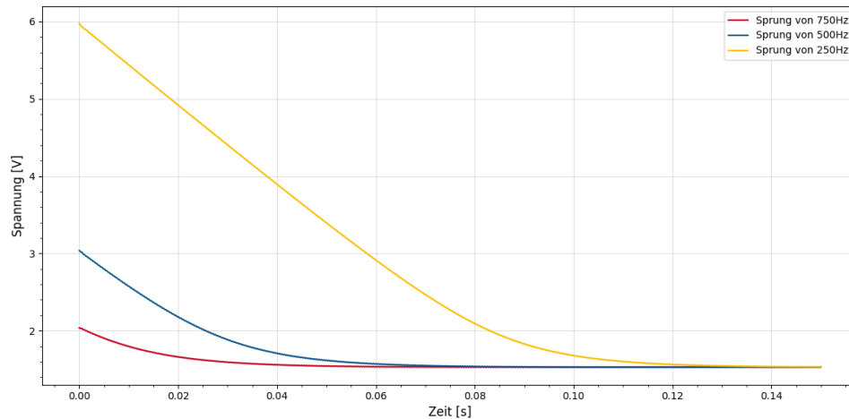
Abbildung 4.7: Validierung der Hypothese zur Einschwingdauer
