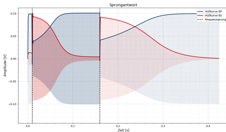
Abbildung 4.6: Amplituden-Einschwingverhalten für Bandpass und Bandsperre
