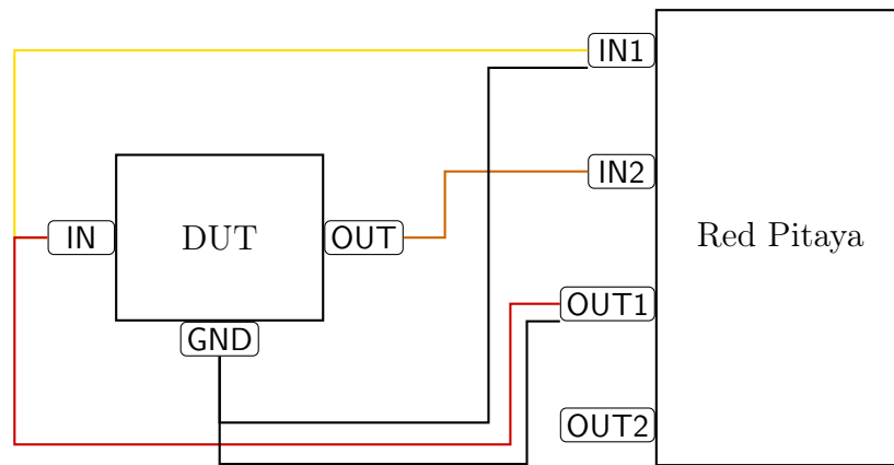
Abbildung 7.1: Messaufbau zur Charakterisierung des DUT mit dem Red Pitaya
