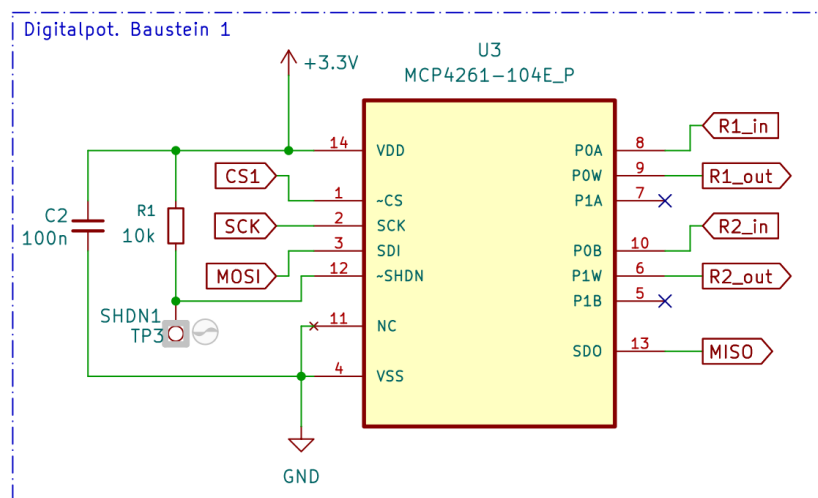
Abbildung 6.4: Verschaltung der Digitalpotentiometer MCP4261
