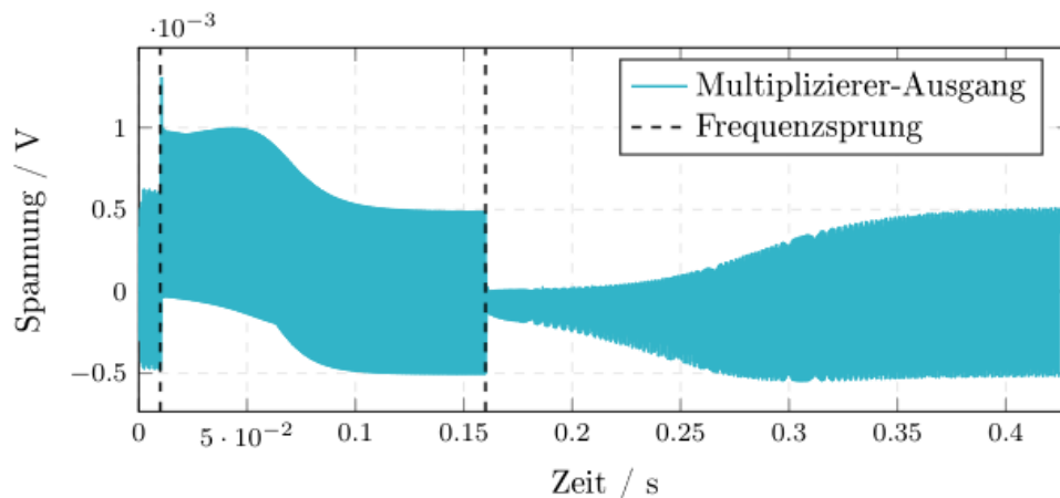
Abbildung 4.2: Signalverlauf am Multiplizierer im Phasendetektor
