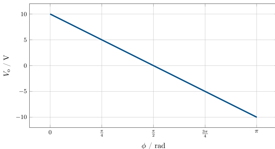
Abbildung 3.10: Phasencharakteristik des Multiplizierers YT_stf_lecture23
