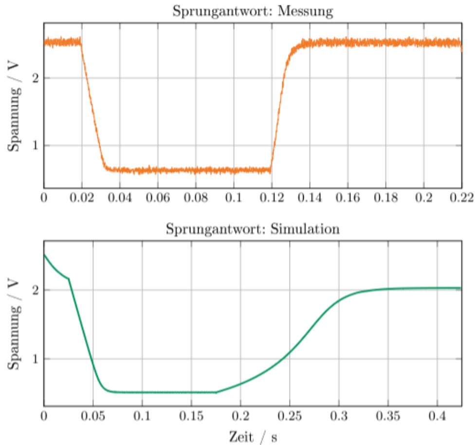
Abbildung 7.3: Verlauf der Steuerspannung V_c
