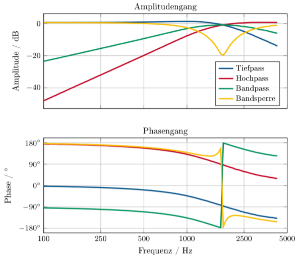
Abbildung 6.3: Amplituden und Phasenverläufe der Filter des VCF
