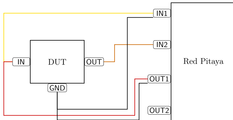
Abbildung 6.1: Messaufbau zur Charakterisierung des DUT mit dem Red Pitaya LabANS
