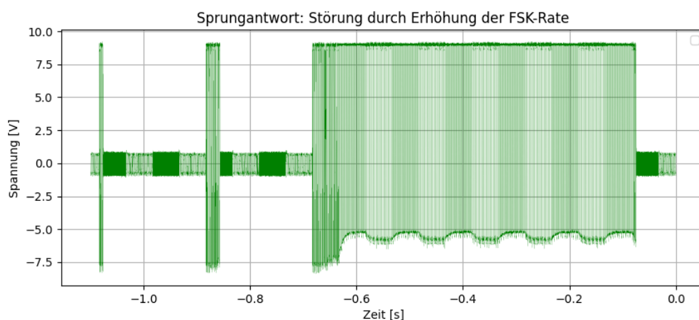
Abbildung 6.6: Bild der Störung
