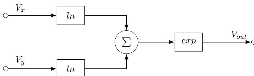
Abbildung 3.6: Funktionelle Realisierung eines Analogmultiplizierers mult_wiki
