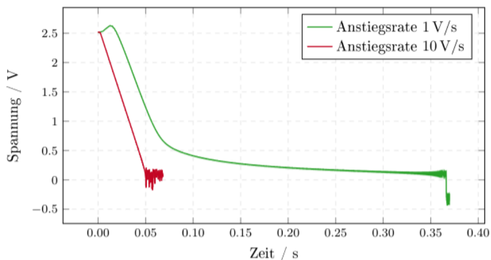
Abbildung 4.8: Vergleich der Steuerspannung bei unterschiedlichen Frequenzanstiegsraten
