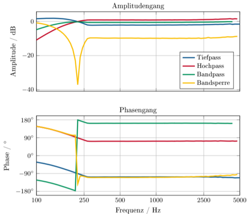
Abbildung 6.2: Amplituden und Phasenverläufe der Filter im Gesamtsystem
