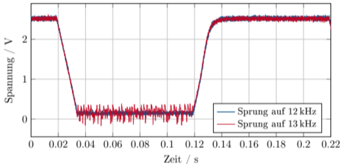
Abbildung 7.9: Verhalten der Steuerspannung an der oberen Filtergrenze
