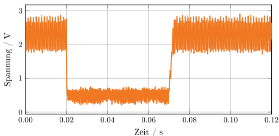
Abbildung 7.2: Einschwingverhalten der Steuerspannung V_c für V_{in_{pp}} = 2\text{ V}
