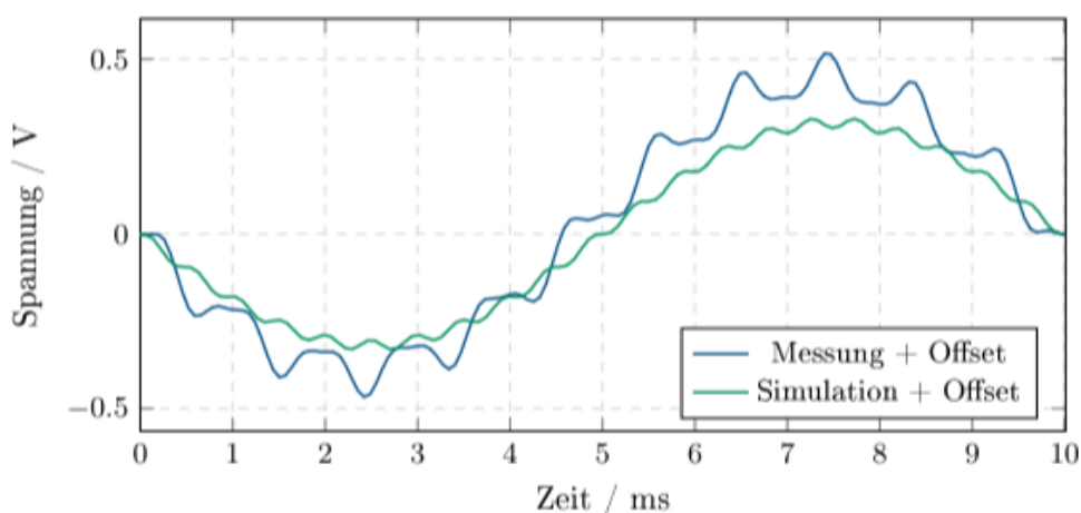
Abbildung 6.5: Ausgangssignal des Phasendetektors (AC-Betrachtung)
