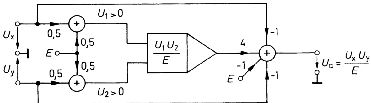
Abbildung 3.7: Vom Einquadranten- zum Vierquadranten-Multiplizierer halbleiter_4Quad
