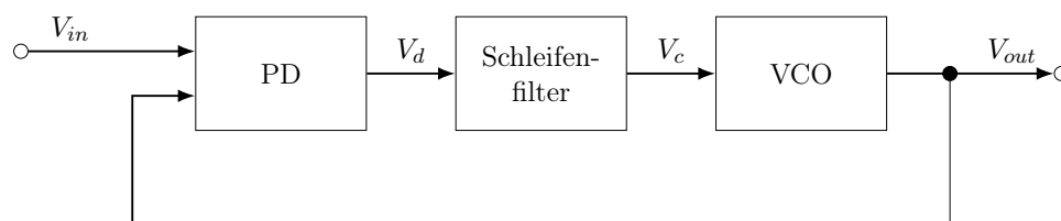
Abbildung 3.4: Einfacher Aufbau eines PLL razaviRF
