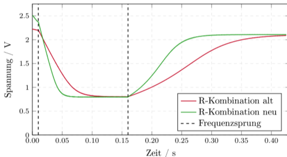
Abbildung 4.7: PD-Ausgang für verschiedene Widerstandskombinationen
