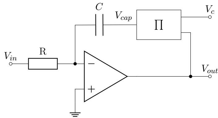
Abbildung 3.17: Teilschaltung: Spannungsgesteuerter Integrator (VCI)
