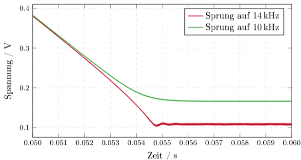
Abbildung 4.9: Einschwingverhalten der Steuerspannung für unterschiedliche Frequenzen
