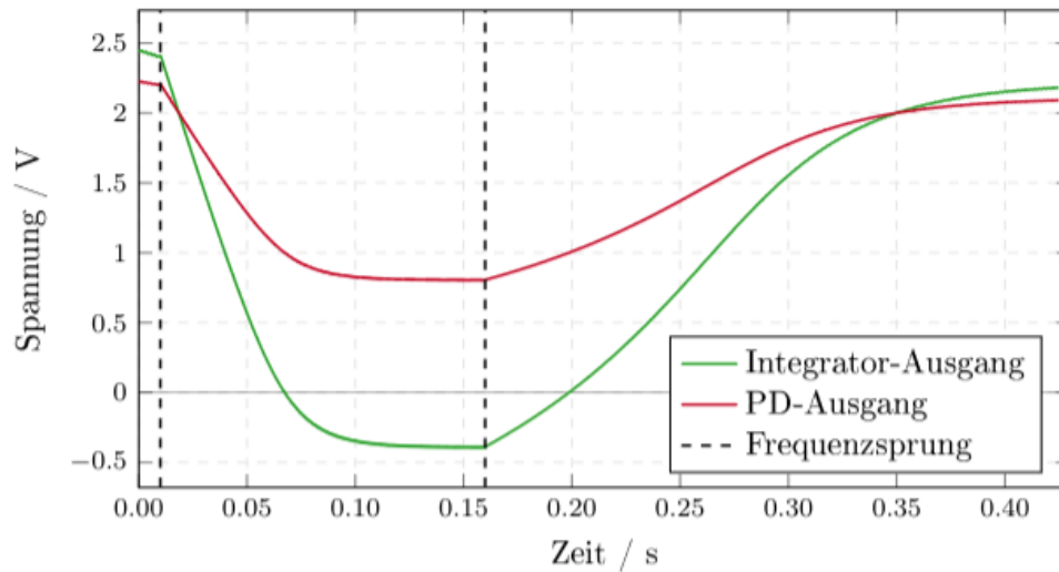
Abbildung 4.6: Spannungsvergleich am Integrator- und Phasendetektorausgang
