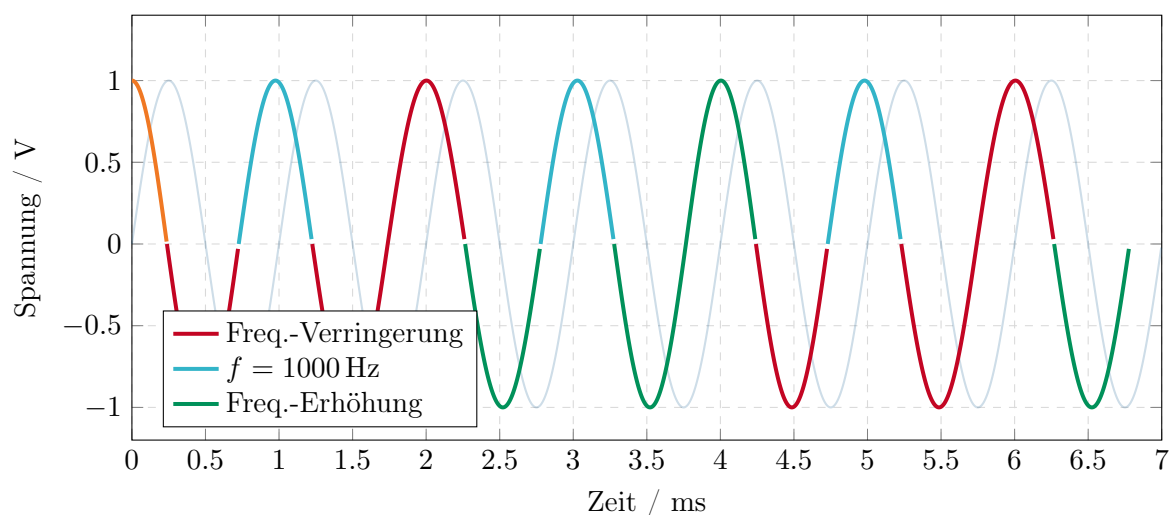
Abbildung 3.20: Signalverhalten bei diskreter Frequenzänderung anhand der Phasenlage
