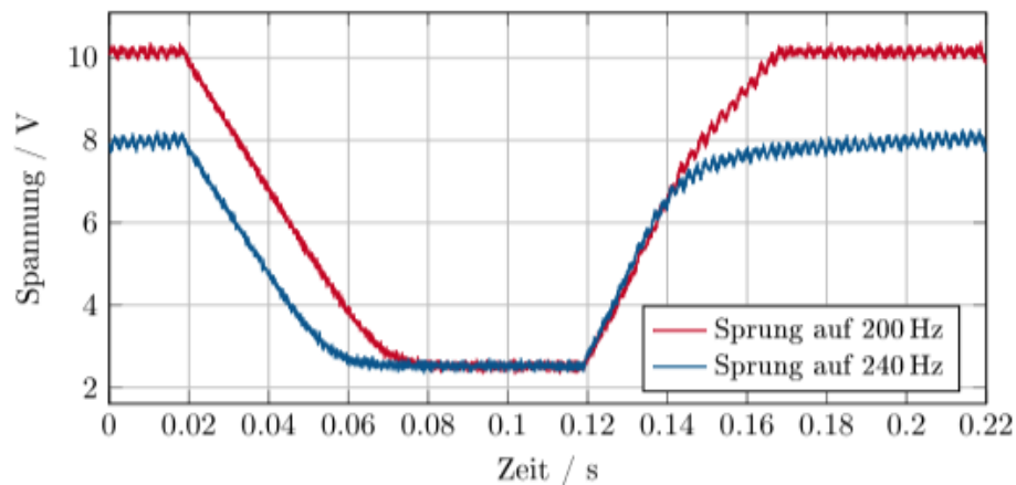
Abbildung 7.8: Verhalten der Steuerspannung an der unteren Filtergrenze
