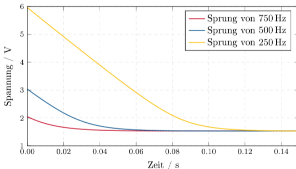
Abbildung 4.5: Validierung der Hypothese zur Einschwingdauer
