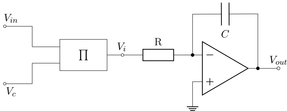
Abbildung 3.19: Vereinfachter Schaltplan zur Herleitung von \omega_0
