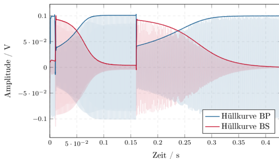
Abbildung 4.4: Amplituden-Einschwingverhalten für Bandpass und Bandsperre
