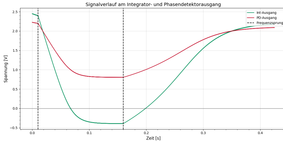
Abbildung 4.6: Spannungsvergleich am Integrator- und Phasendetektorausgang
