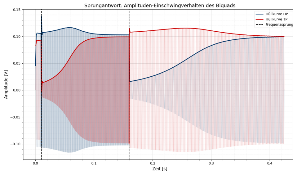
Abbildung 5.2: Amplituden-Einschwingverhalten des Biquads für Hoch- und Tiefpass
