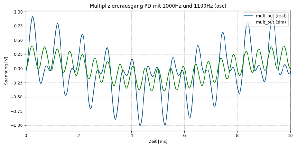
Abbildung 7.2: Ausgangssignal des Multiplizierers innerhalb des PD
