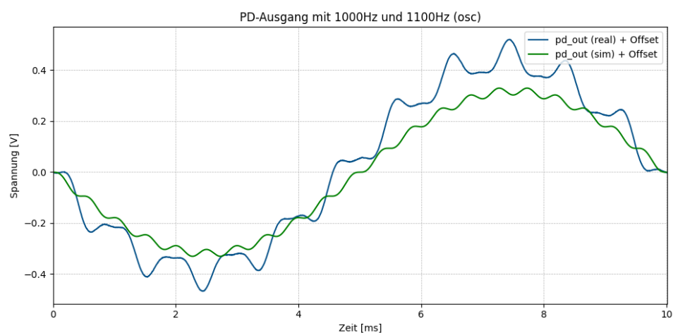
Abbildung 7.3: Ausgangssignal des Phasendetektors
