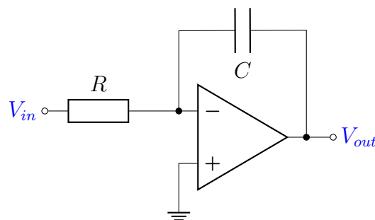
Abbildung 3.2: Invertierender Integrator
