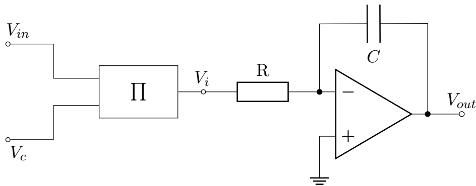
Abbildung 3.19: Vereinfachter Schaltplan zur Herleitung von \omega_0
