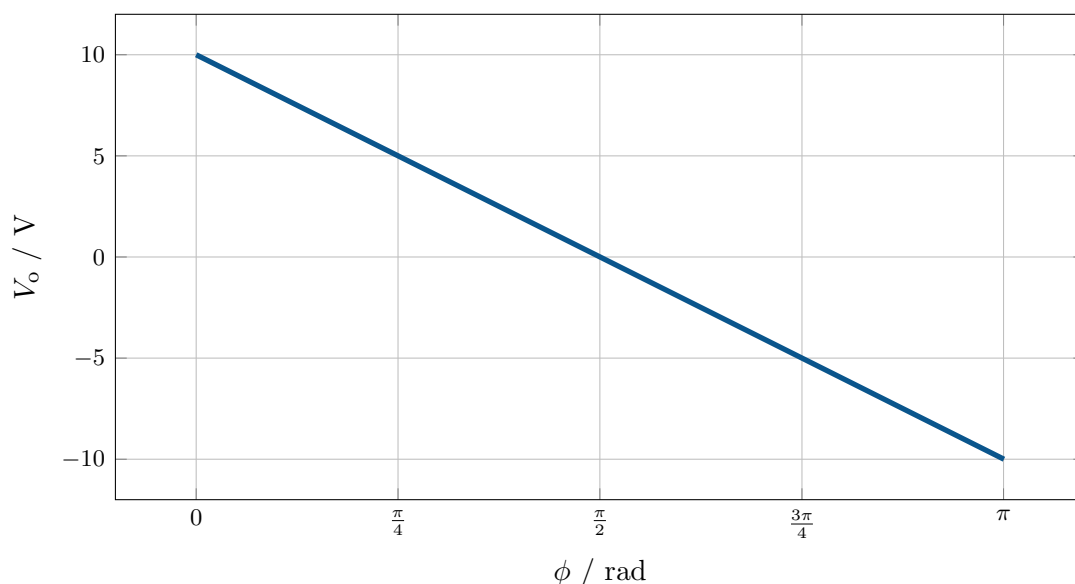
Abbildung 3.10: Phasencharakteristik des Multiplizierers [10]
