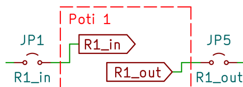
Abbildung 5.3: Darstellung der Ein- und Ausgänge der Digitalpotentiometer
