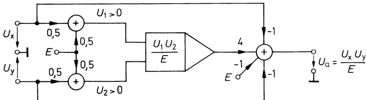
Abbildung 3.7: Vom Einquadranten- zum Vierquadranten-Multiplizierer[4]
