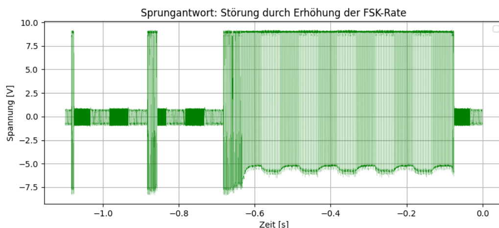
Abbildung 6.6: Bild der Störung
