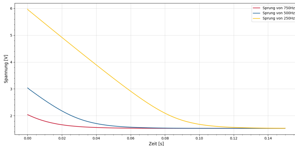
Abbildung 4.5: Validierung der Hypothese zur Einschwingdauer
