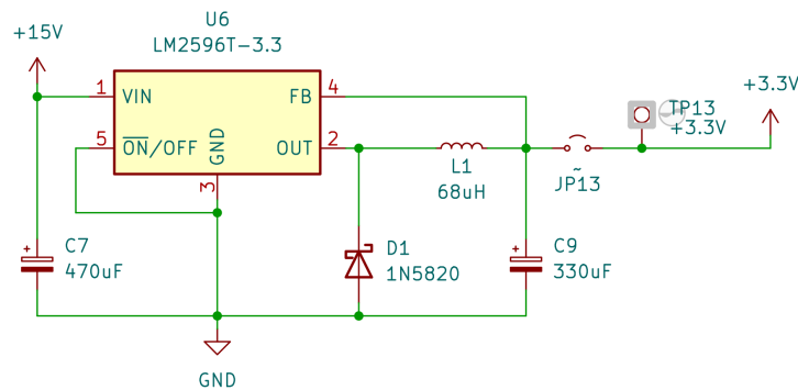
Abbildung 5.7: Aufbau des Buck-Converters
