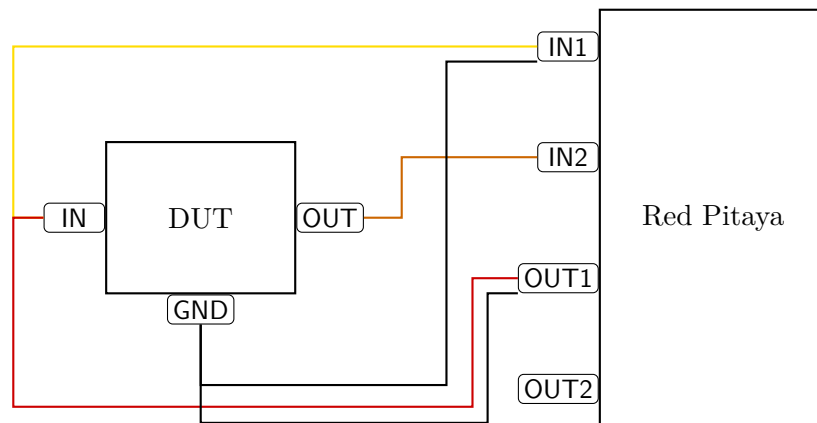
Abbildung 6.1: Messaufbau zur Charakterisierung des DUT mit dem Red Pitaya [3]
