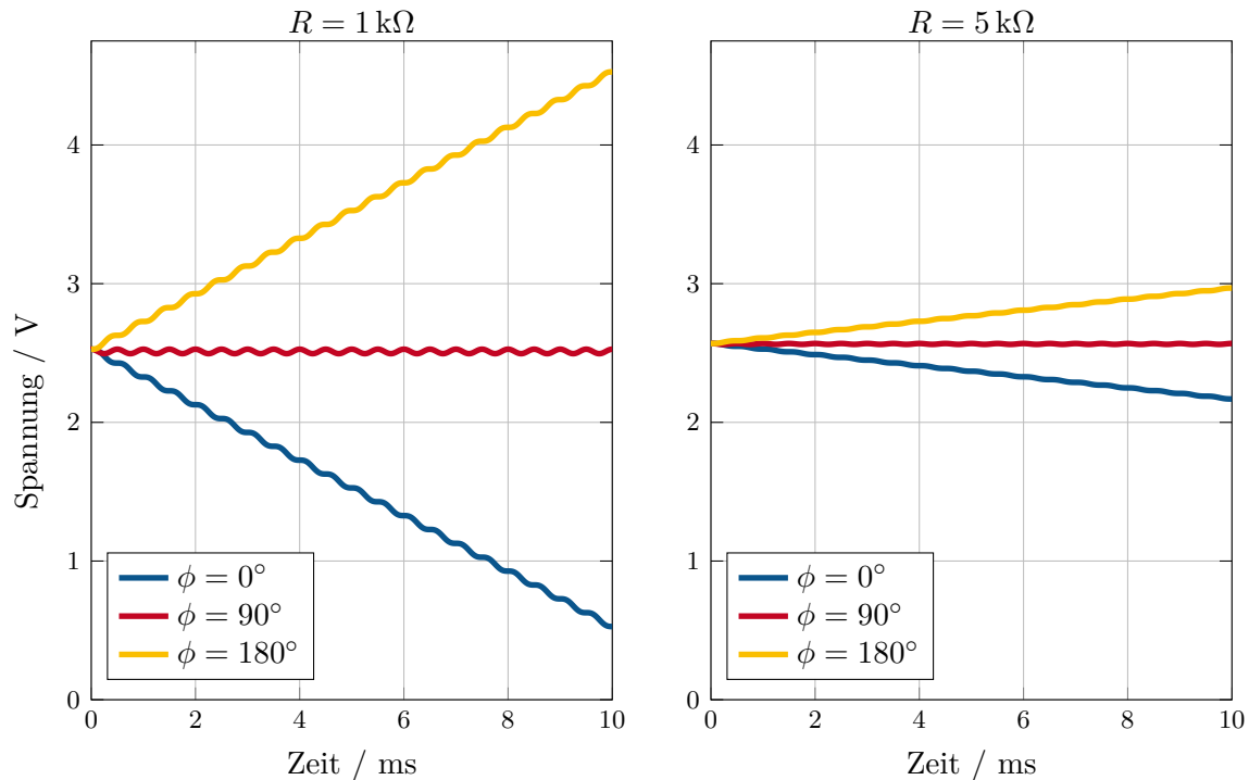
Abbildung 3.14: Signalverhalten bei unterschiedlicher Verschaltung des Integrators
