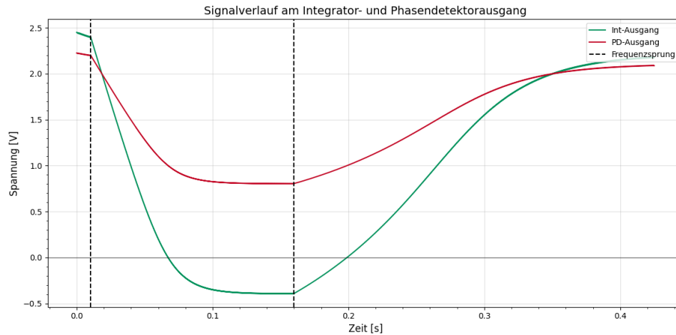
Abbildung 4.6: Spannungsvergleich am Integrator- und Phasendetektorausgang
