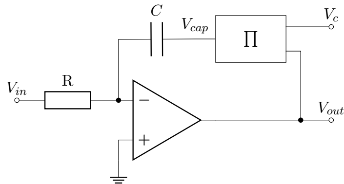
Abbildung 3.17: Teilschaltung: Spannungsgesteuerter Integrator (VCI)
