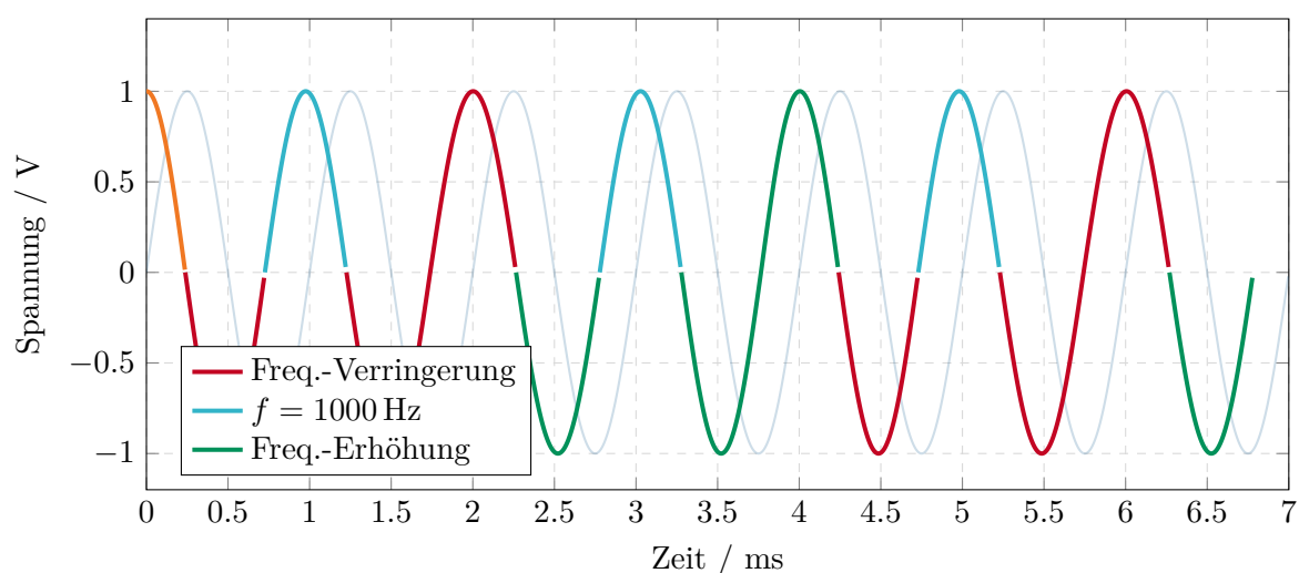
Abbildung 3.20: Signalverhalten bei diskreter Frequenzänderung anhand der Phasenlage
