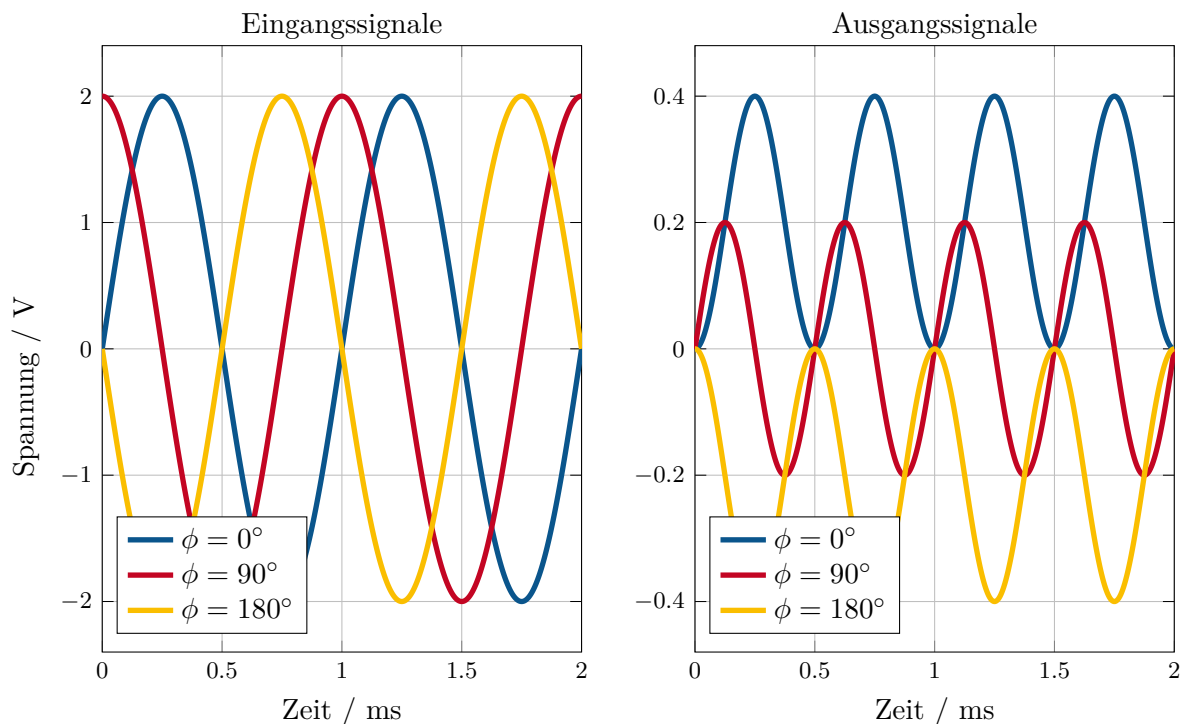
Abbildung 3.13: Signalverhalten bei unterschiedlichen Phasenlagen zwischen den Eingangssignalen X_1 und Y_1
