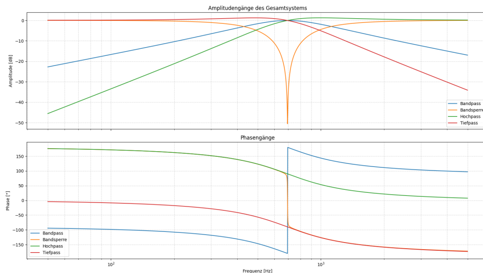
Abbildung 4.1: Kleinsignalanalyse des Gesamtsystems
