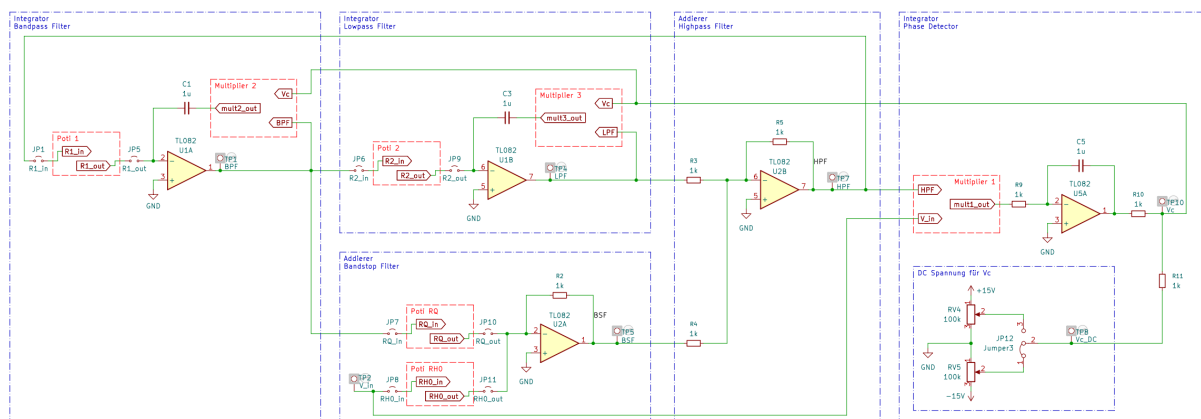
Abbildung 5.1: Darstellung des VCF ohne Peripherie
