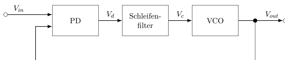
Abbildung 3.4: Einfacher Aufbau eines PLL [8]
