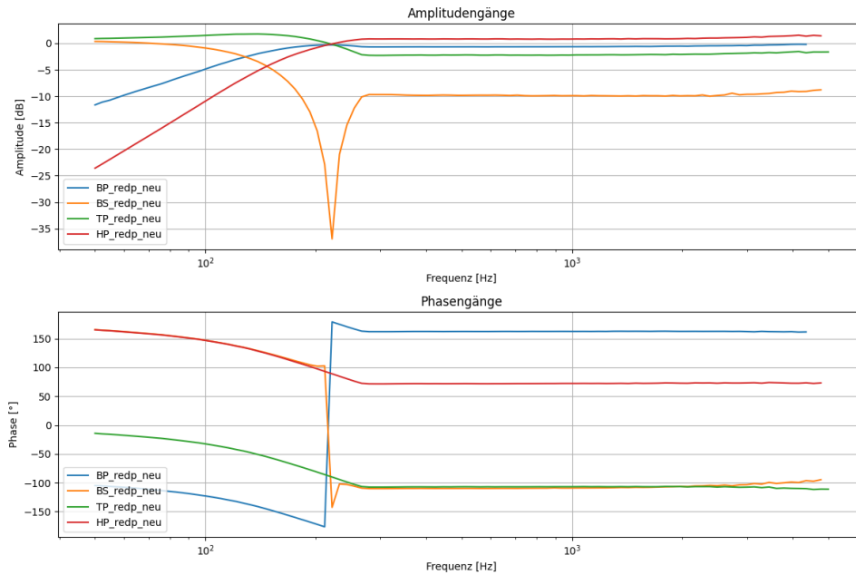
Abbildung 6.2: Amplituden und Phasenverläufe der Filter im Gesamtsystem
