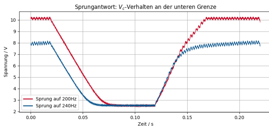
Abbildung 7.8: Verhalten der Steuerspannung an der unteren Filtergrenze
