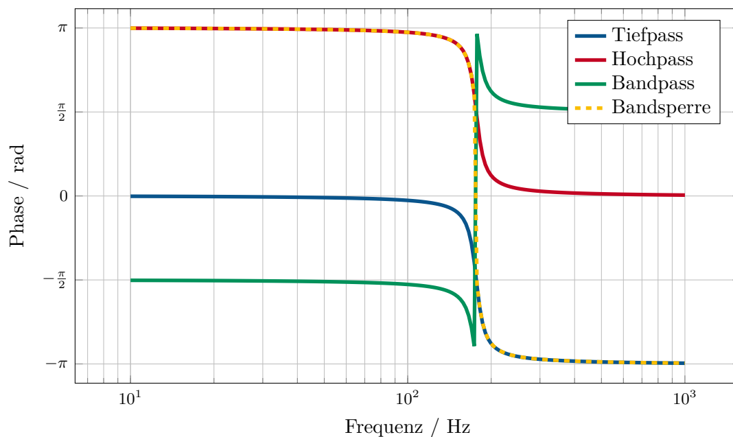
Abbildung 3.11: Phasengang der vier Ausgänge des Biquads
