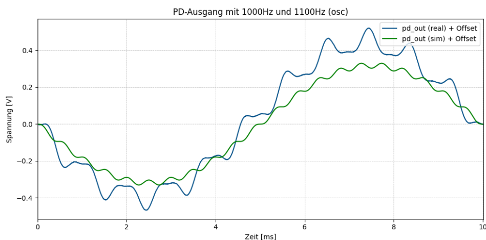
Abbildung 6.5: Ausgangssignal des Phasendetektors (AC-Betrachtung)
