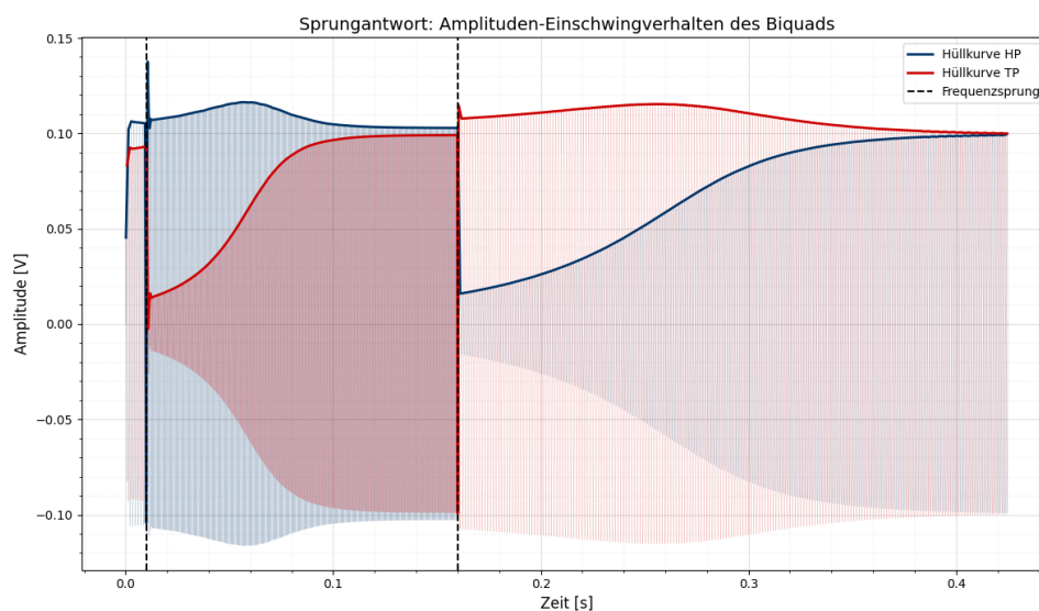
Abbildung 4.3: Amplituden-Einschwingverhalten des Biquads für Hoch- und Tiefpass
