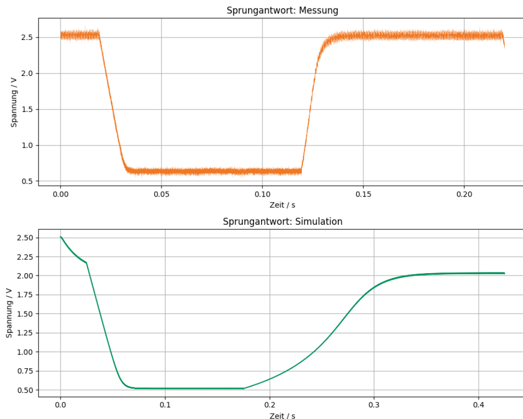
Abbildung 7.3: Verlauf der Steuerspannung V_c
