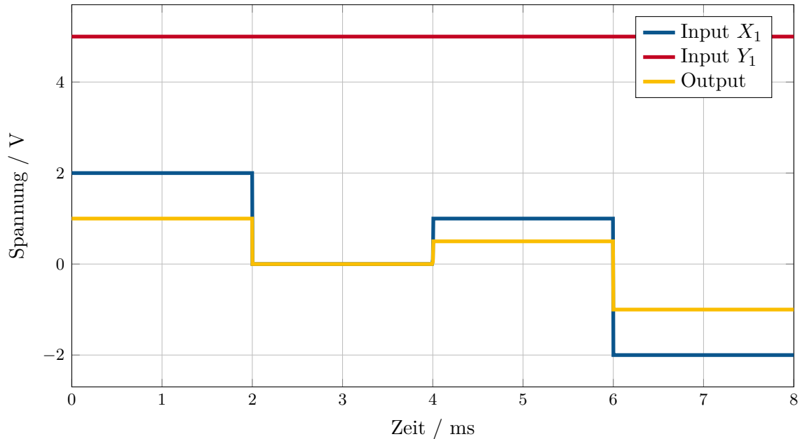
Abbildung 3.8: Demonstration des analogen Multiplizierers mit Gleichspannungen
