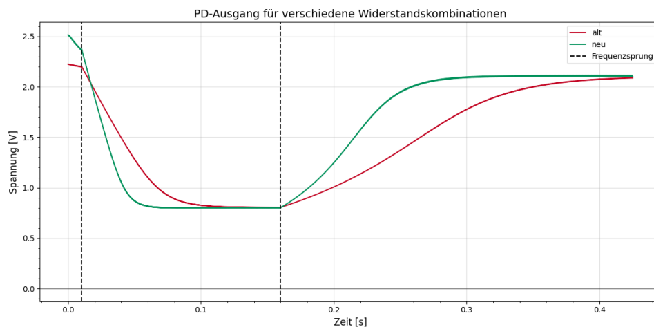
Abbildung 4.7: PD-Ausgang für verschiedene Widerstandskombinationen
