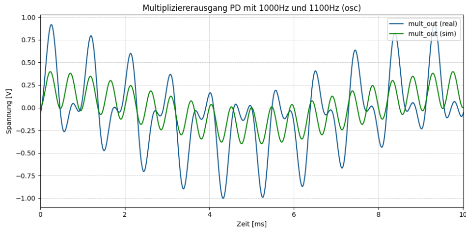
Abbildung 6.4: Ausgangssignal des Multiplizierers im Phasendetektor
