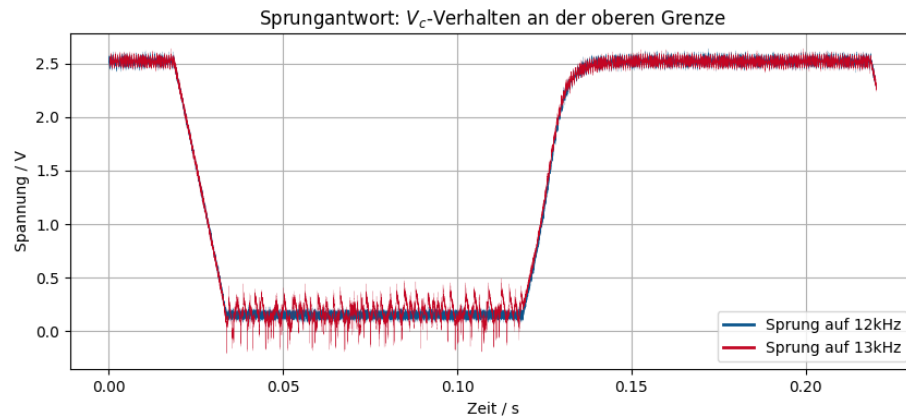
Abbildung 7.9: Verhalten der Steuerspannung an der oberen Filtergrenze
