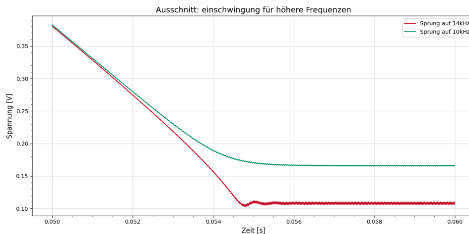
Abbildung 4.9: Einschwingverhalten der Steuerspannung für unterschiedliche Frequenzen
