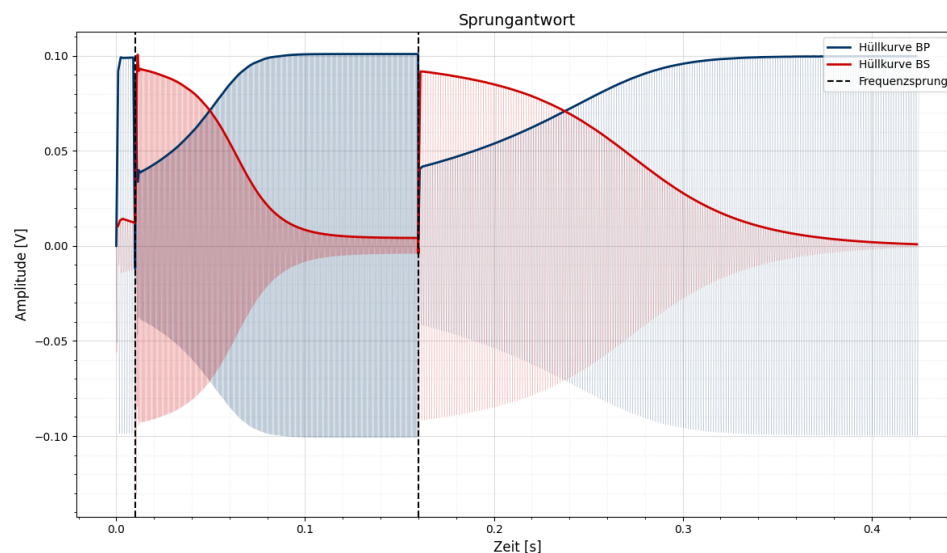
Abbildung 4.4: Amplituden-Einschwingverhalten für Bandpass und Bandsperre
