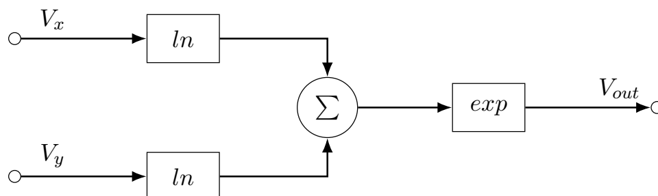
Abbildung 3.6: Funktionelle Realisierung eines Analogmultiplizierers [9]
