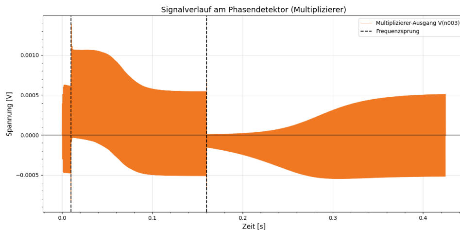
Abbildung 4.2: Signalverlauf am Multiplizierer im Phasendetektor
