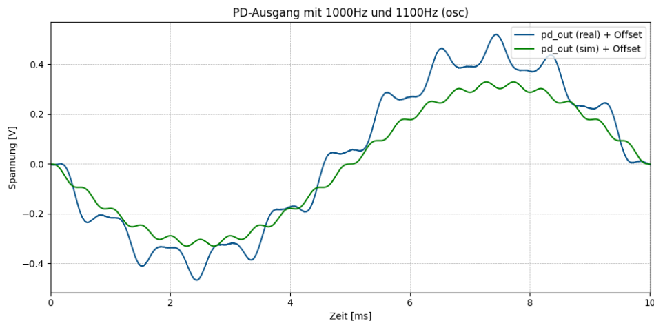
Abbildung 1.3: Ausgangssignal des Phasendetektors
