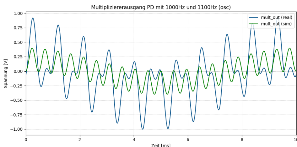
Abbildung 1.2: Ausgangssignal des Multiplizierers innerhalb des PD
