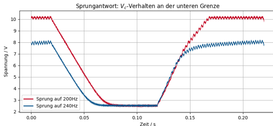
Abbildung 1.8: Verhalten der Steuerspannung an der unteren Filtergrenze
