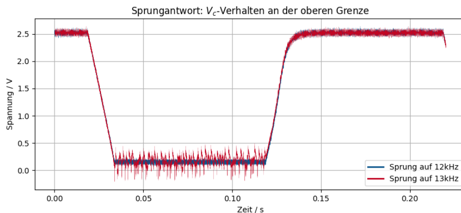
Abbildung 1.9: Verhalten der Steuerspannung an der oberen Filtergrenze
