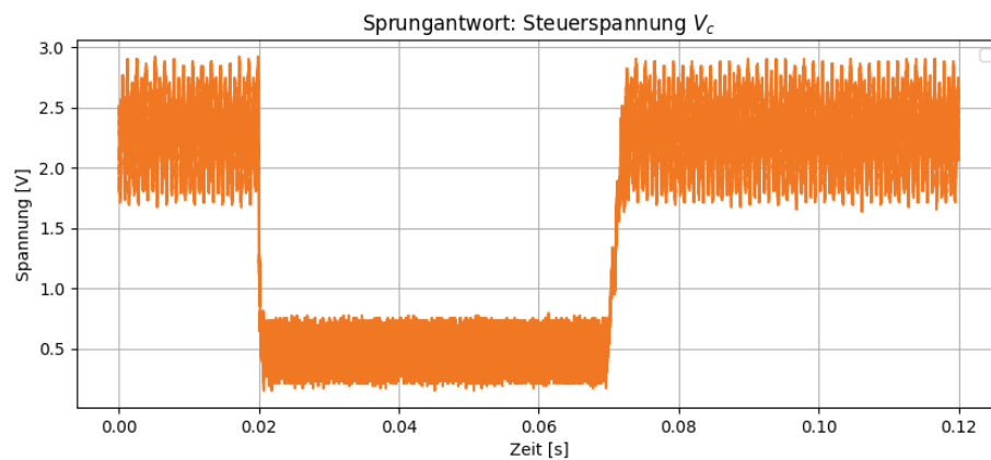
Abbildung 1.2: Einschwingverhalten der Steuerspannung V_c für V_{inpp} = 2\text{ V}
