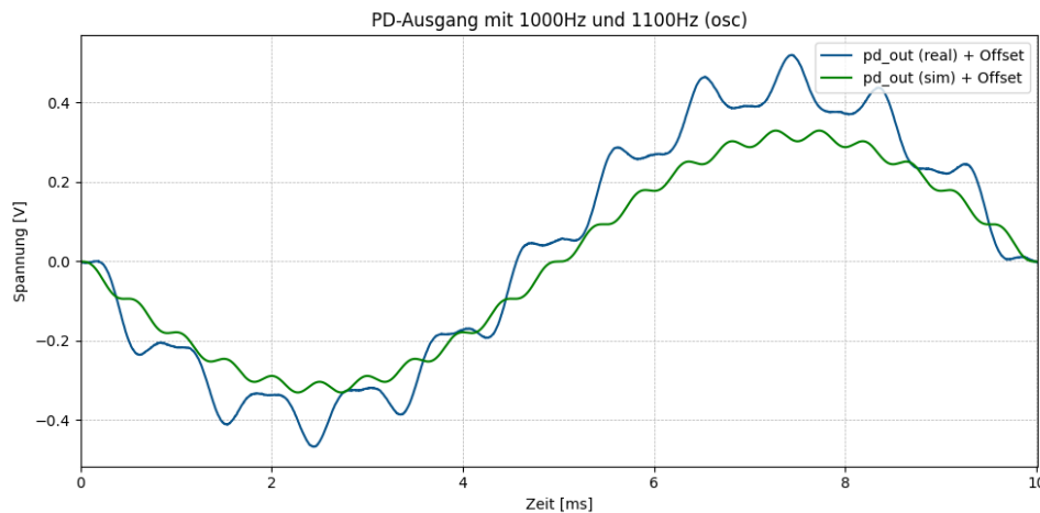
Abbildung 1.5: Ausgangssignal des Phasendetektors (AC-Betrachtung)
