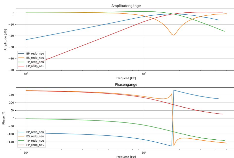
Abbildung 1.3: Amplituden und Phasenverläufe der Filter des VCF
