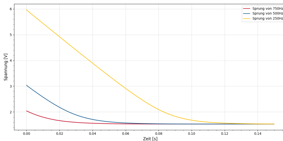
Abbildung 4.5: Validierung der Hypothese zur Einschwingdauer
