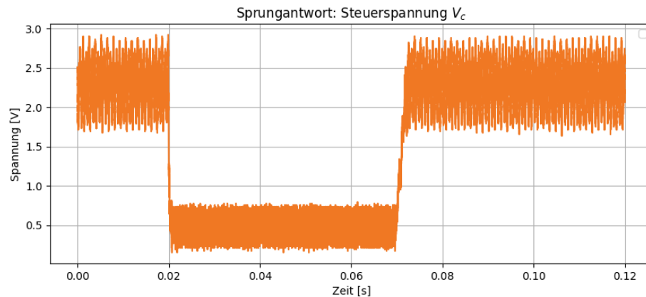
Abbildung 7.2: Einschwingverhalten der Steuerspannung V_c für V_{inpp} = 2\text{ V}
