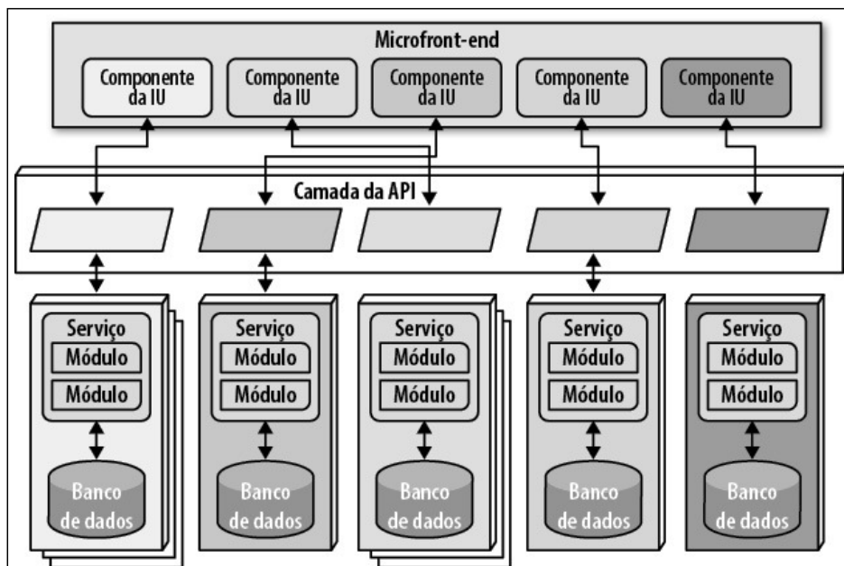
Figura 17-6. Padrão microfront-end em microserviços
