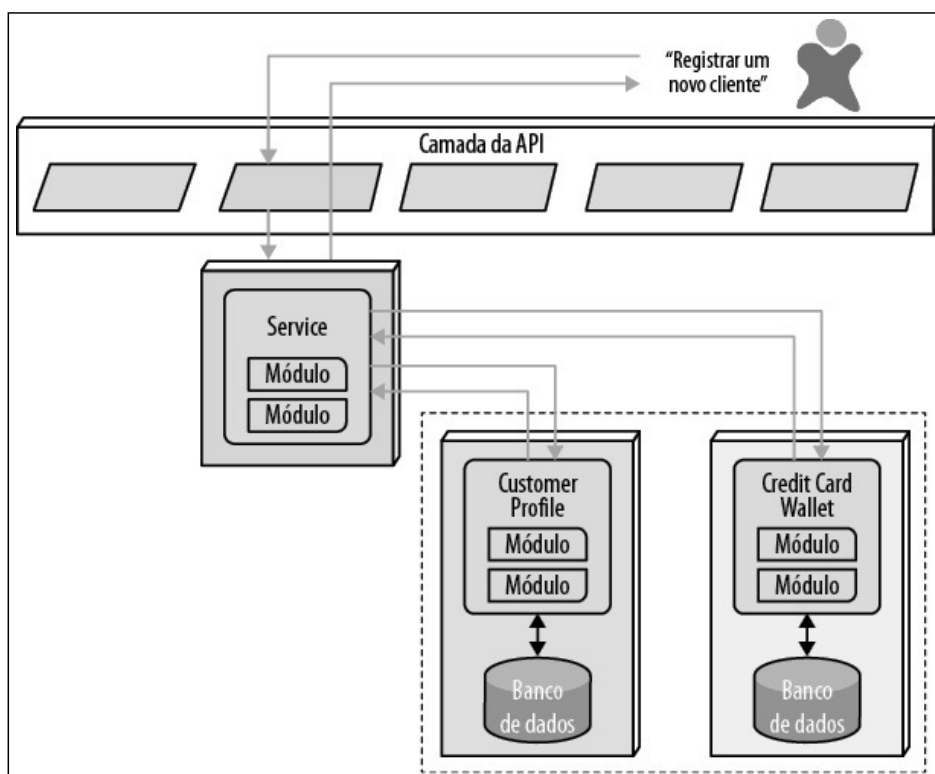
Figura 17-11. Padrão saga na arquitetura de microserviços
