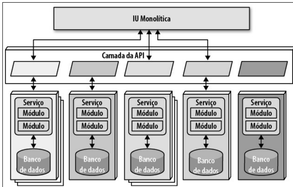
Figura 17-5. Arquitetura de microserviços com uma IU monolítica
