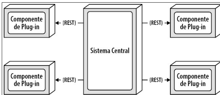
Figura 12-6. Acesso do plug-in remoto usando REST
