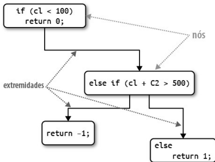
Figura 6-1. Complexidade Ciclomática para a função de decisão
