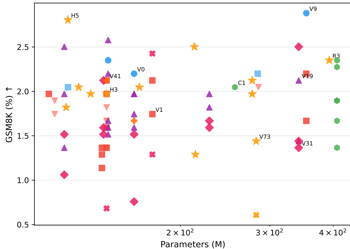
GSM8K vs. Parameters
