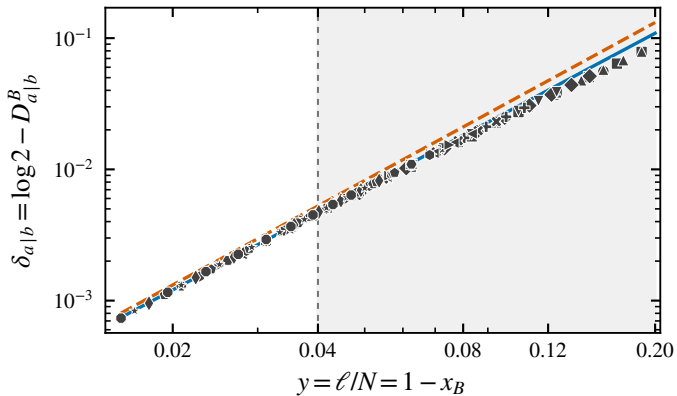
(f) 3s,s|ss
