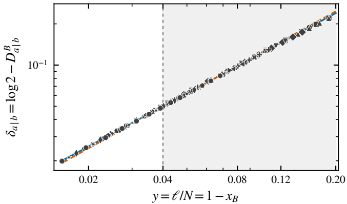
(d) 3s,s|00
