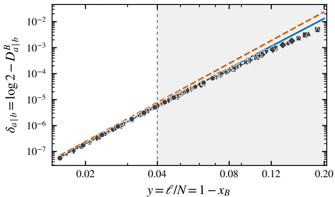
(f) 3s,s|ss
