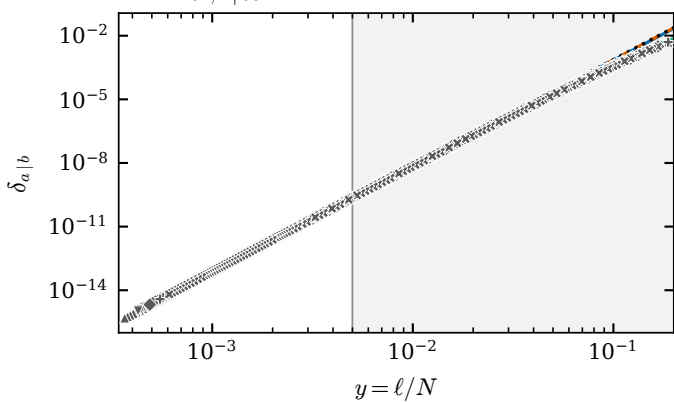
(f) \delta_{3s,s|ss}
