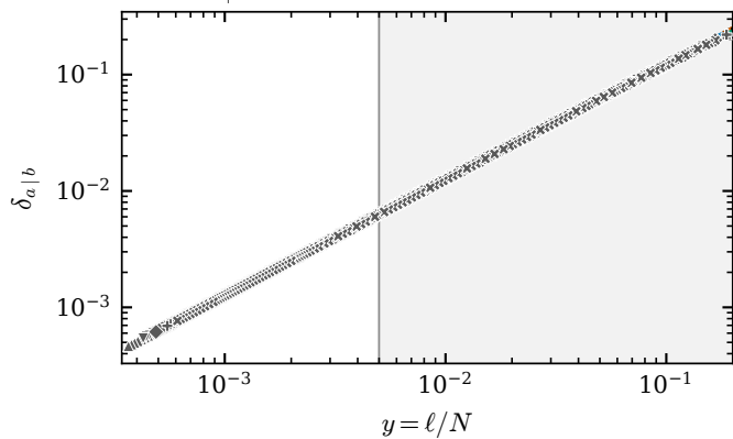
(d) \delta_{3s,s|00}
