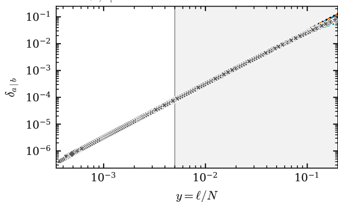
(f) \delta_{3s,s|ss}
