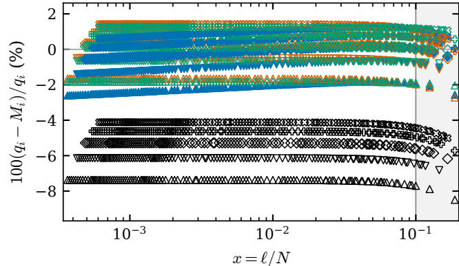
(d) D_{3s,s|00}^A
