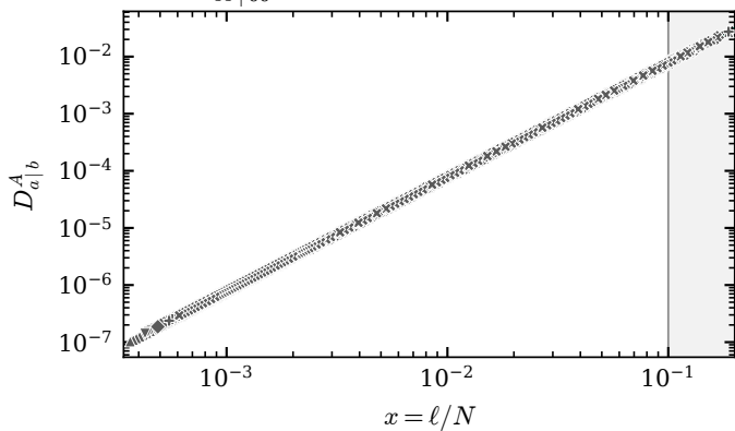
(d) D_{3s,s|00}^A
