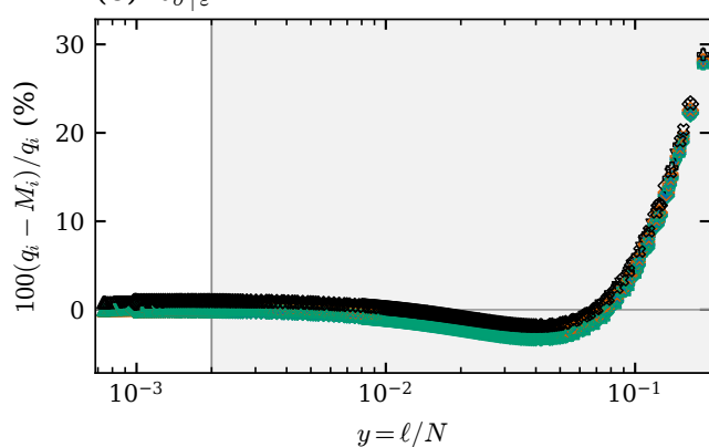
(e) \delta_{\sigma|\varepsilon}
