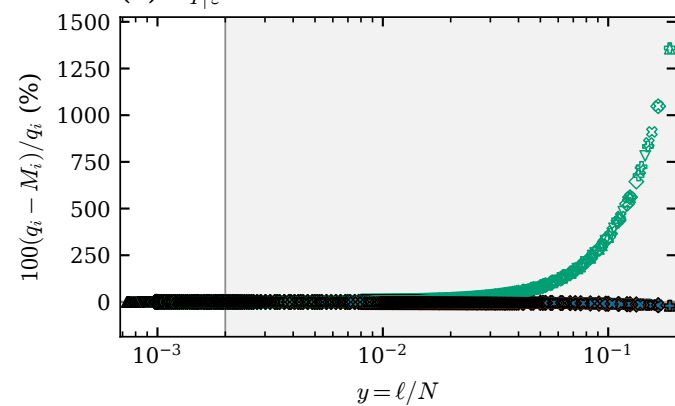
(e) \delta_{\sigma|\varepsilon}
