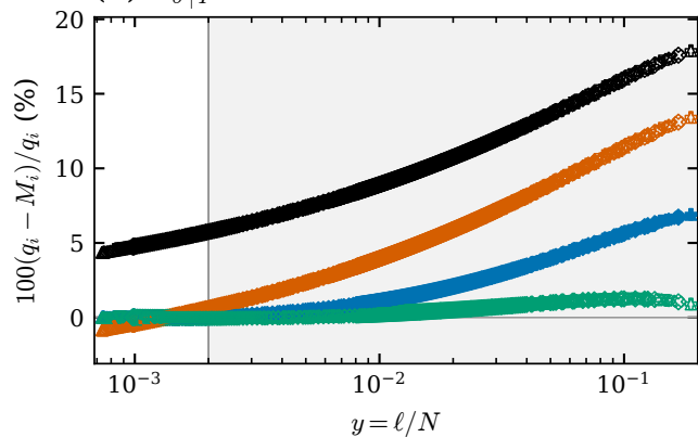
(d) \delta_{\varepsilon|I}
