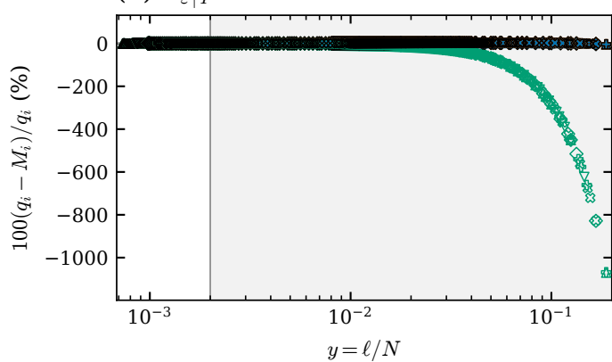
(f) \delta_{\varepsilon|\sigma}
