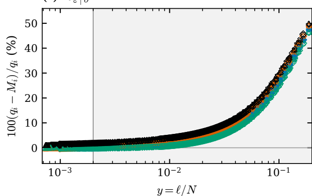
(f) \delta_{\varepsilon|\sigma}
