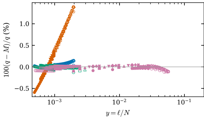
(d) \varepsilon | I
