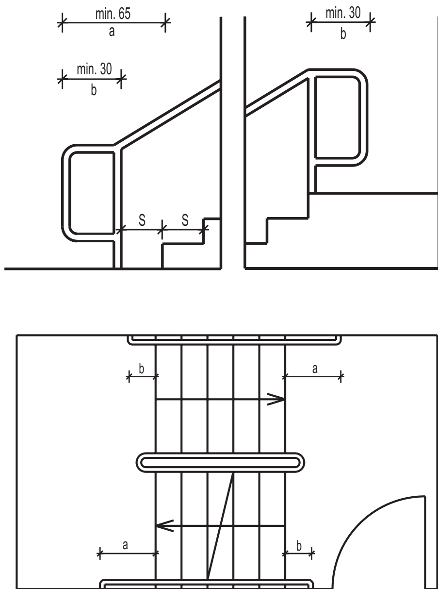
Rys. 5. Komunikacja pionowa. Schody i umieszczanie poręczy.
