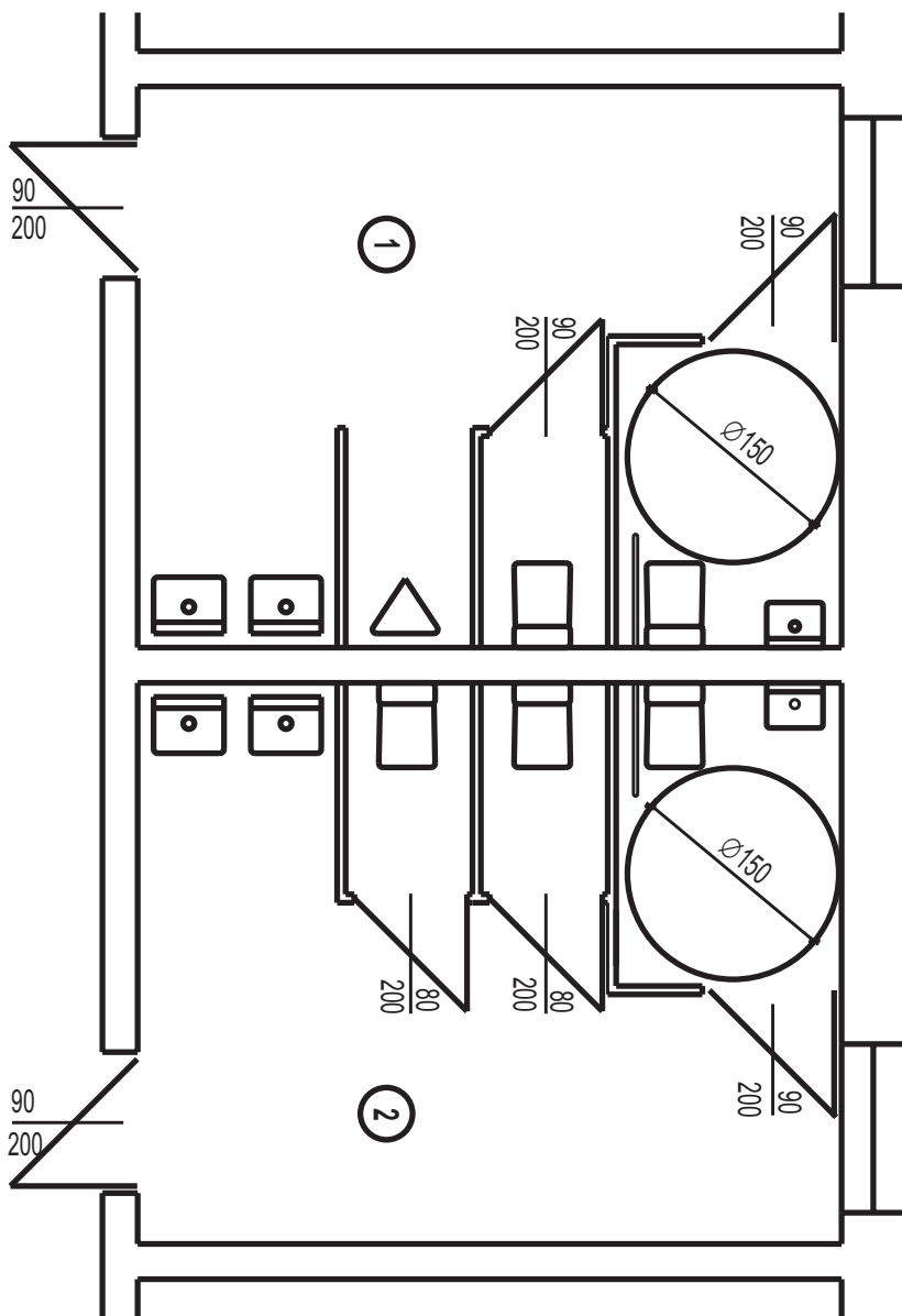
Rys. 9. Pomieszczenie higieniczno-sanitarne ogólnodostępne z wydzielonymi kabinami dla osób niepełnosprawnych w zespole męskim i damskim: 1 – zespół męski, 2 – zespół damski, 3 – kabiny dla osób niepełnosprawnych z dodatkowym wyposażeniem w uchwyty.
