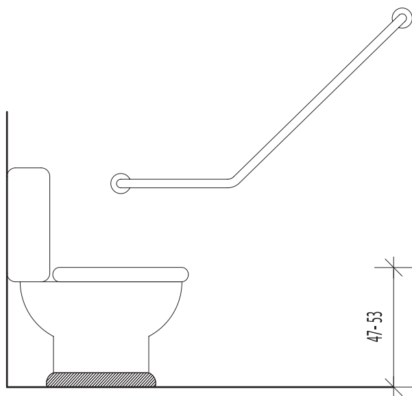
Rys. 11. Uchwyty przy misce ustępowej i sposoby jej podwyższania.
