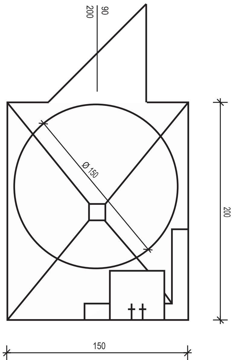
Rys. 15. Przykład rzutu kabiny natryskowej z wyprofilowanym w posadzce spadkiem kratki ściekowej oraz dodatkowym wyposażeniem w uchwyty i siedzisko prysznicowe.
