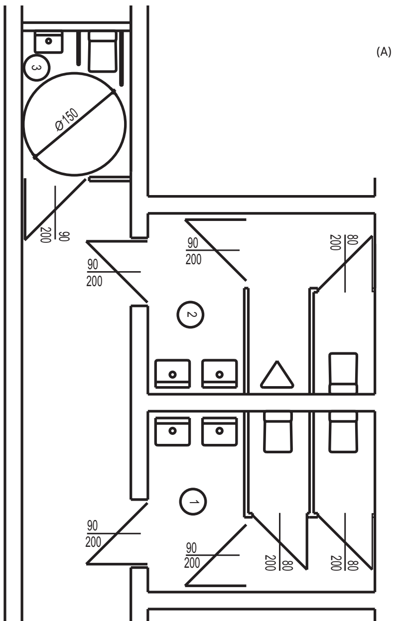
Rys. 8. Pomieszczenie higieniczno-sanitarne ogólnodostępne z wydzieloną kabiną dla osób niepełnosprawnych obojga płci: A) dostępne z przedsionka: 1 – zespół męski, 2 – zespół damski, 3 – kabina dla osób niepełnosprawnych z dodatkowym wyposażeniem w uchwyt.
