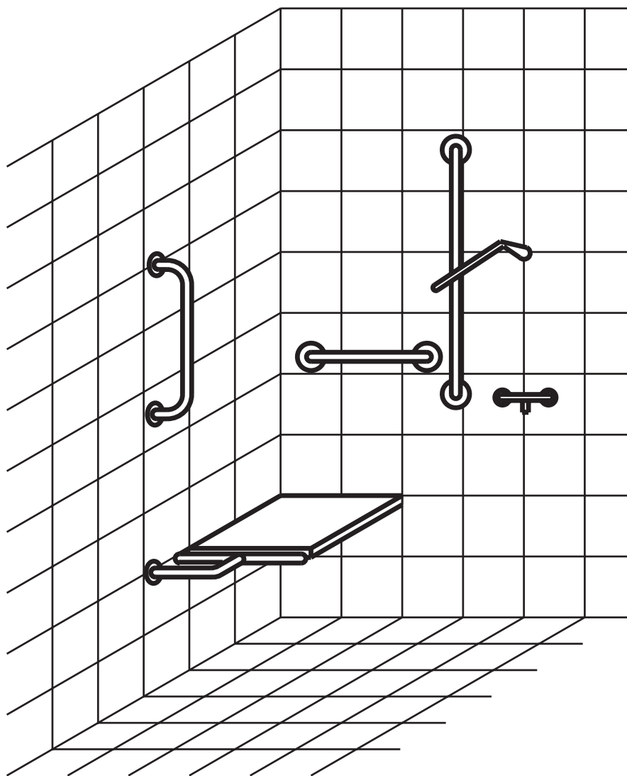
Rys. 13. Pomieszczenia higieniczno-sanitarne. Elementy wyposażenia: natryski, umywalnie.
