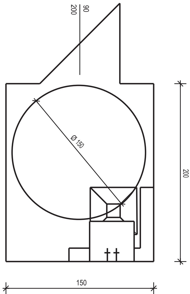
Rys. 16. Przykład rzutu kabiny natryskowej z zastosowaniem bezpośredniego brodzika, uchwytów i siedziska prysznicowego.
