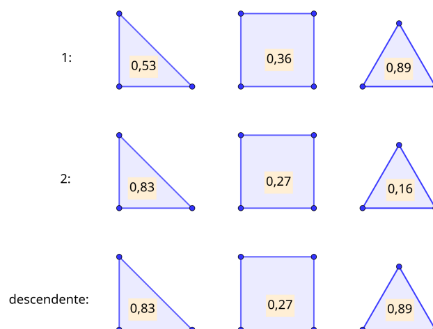
Figura 14 – Cruzamento entre indivíduos 1 e 2 gerando um descendente 3.
