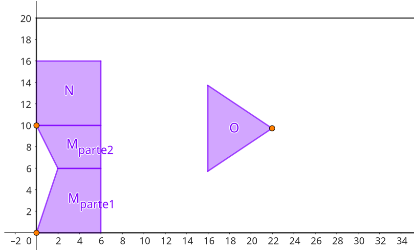
Figura 7 – Polígonos M e N alocados na faixa e O aguardando alocação.
