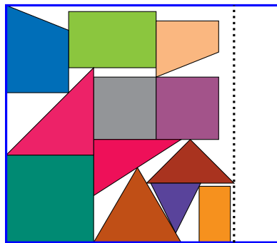
Figura 16 – Melhor resultado da instância fu pela BL (comprimento 36,46), obtido pela BL_{21} .
