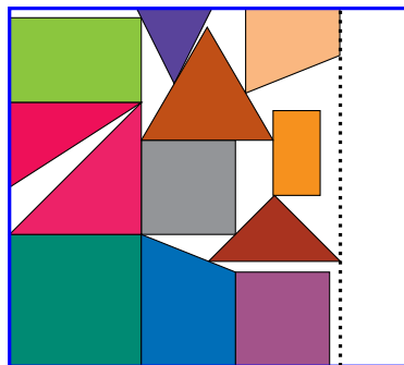
Figura 18 – Melhor resultado da instância fu (comprimento 35,14), obtido pela BRKGA .
