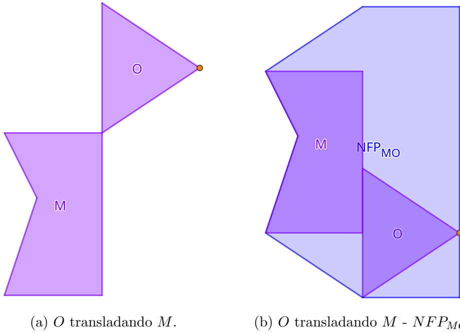
Figura 3 – O polígono O sendo transladado ao redor de M e o caminho feito pelo seu ponto de referência (em laranja) resultando no NFP_{MO} .
