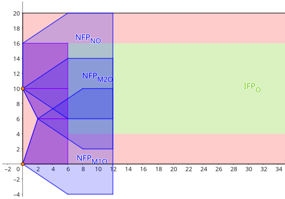
Figura 8 – Polígonos M e N , com os respectivos NFPs em relação a O (note que os NFPs estão posicionados para encaixar perfeitamente com o polígono fixo referente a ele). As intersecções gerarão os possíveis pontos para alocar o ponto de referência de O .
