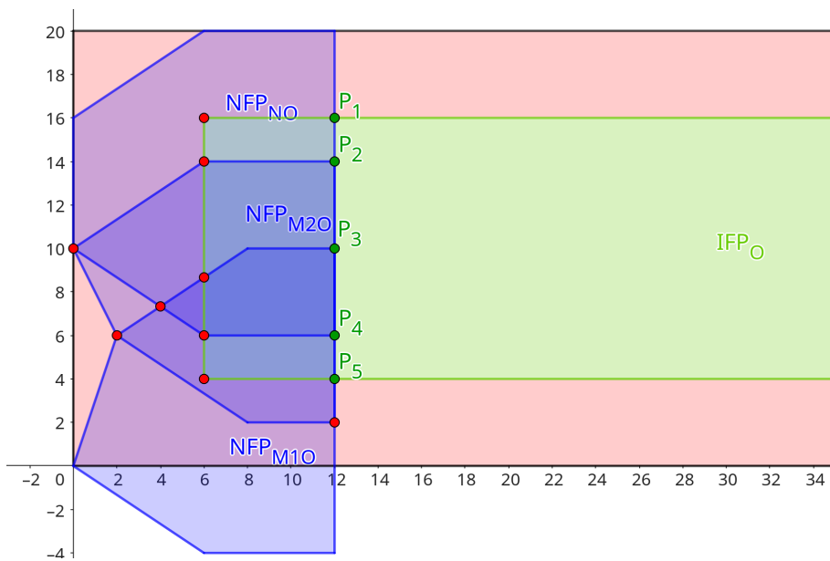
Figura 9 – NFP_{M_1O} , NFP_{M_2O} , NFP_{NO} e os pontos de intersecção entre todos e o IFP_O , onde os pontos em vermelho são posições proibidas e os em verde são posições viáveis.
