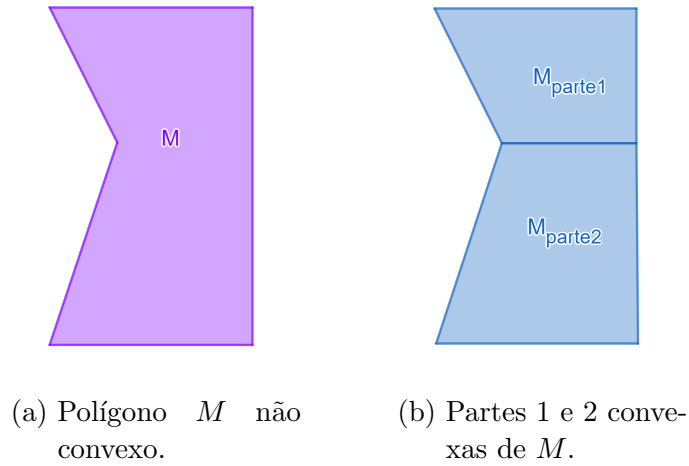
Figura 4 – Polígono M separado em duas partes por não ser convexo.
