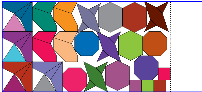
Figura 20 – Melhor resultado da instância blaze1 (comprimento 27,87), obtido pela BRKGA .
