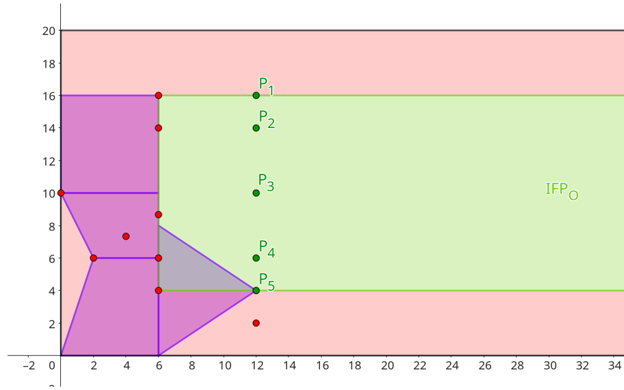
Figura 10 – Todos os pontos de intersecção de O e a posição final onde foi alocado ( P_5 ).
