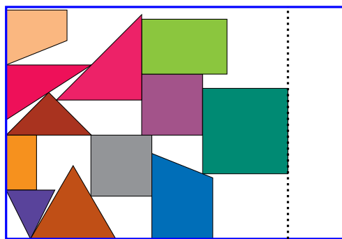
Figura 17 – Pior resultado da instância fu (comprimento 46,25), obtido pela BL_{12} .
