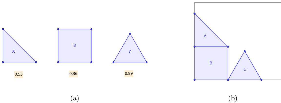
Figura 13 – Chaves do segundo indivíduo geradas em (a) e então sua alocação seguindo a BL após ordenar tais chaves, em (b).
