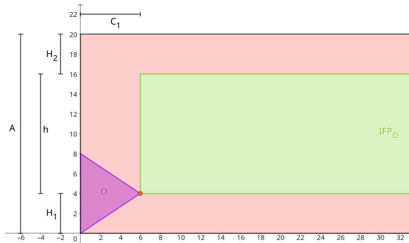
Figura 2 – A área em verde é o IFP do polígono O .
