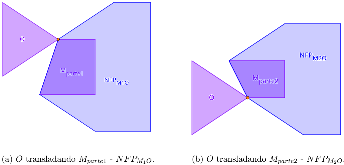
Figura 5 – Montagem das duas partes do NFP_{MO} .
