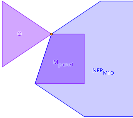
(a) O trasladando M_{parte1} - NFP_{M_1O} .
