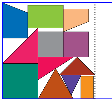
Figura 16: Melhor resultado da instância fu pela BL (comprimento 36,46), obtido pela BL_{21} .
