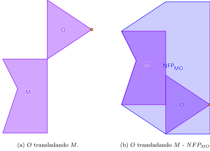
Figura 3: O polígono O sendo transladado ao redor de M e o caminho feito pelo seu ponto de referência (em laranja) resultando no NFP_{MO} .
