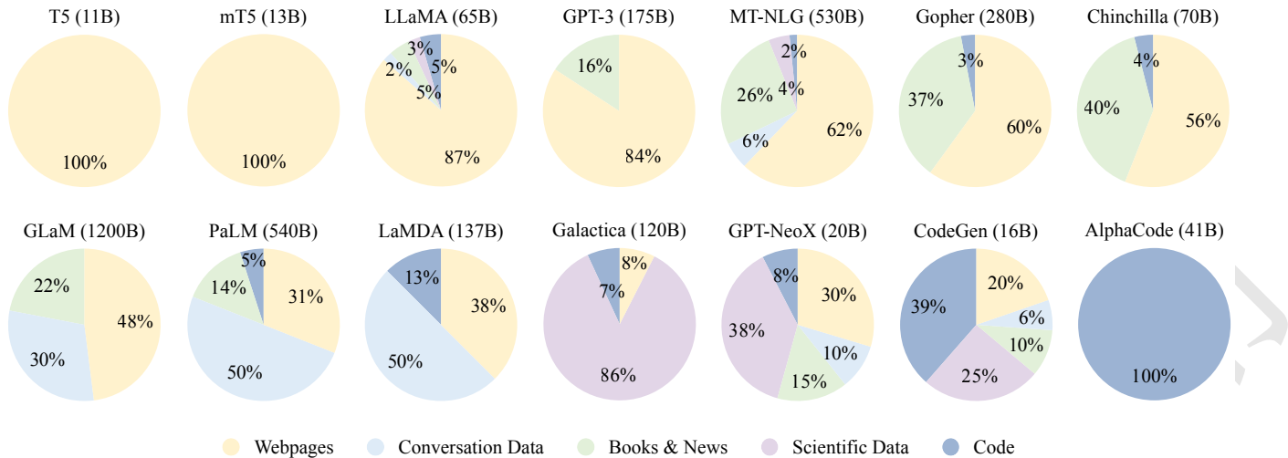
图 2. 现有大语言模型预训练数据中各种数据源的比率。
