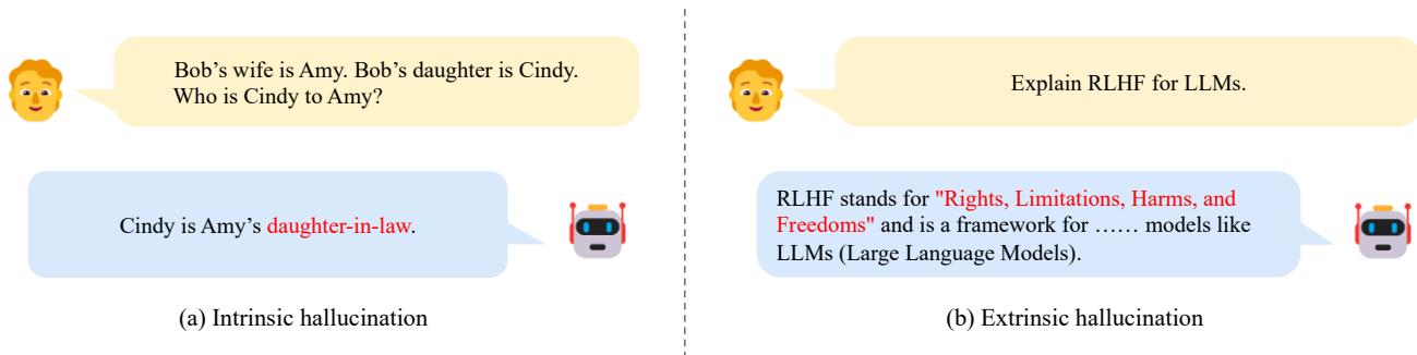
图 7. 一个开放大语言模型的内在和外在幻觉的例子（访问日期：2023 年 3 月 19 日）。作为内在幻觉的例子，大语言模型对 Cindy 和 Amy 之间的关系给出了错误的判断，这与输入相矛盾。对于外在的幻觉，在这个例子中，大语言模型似乎对 RLHF（从人类反馈中强化学习）的含义有不正确的理解，尽管它能正确理解 LLM 的含义（在本例中）。
