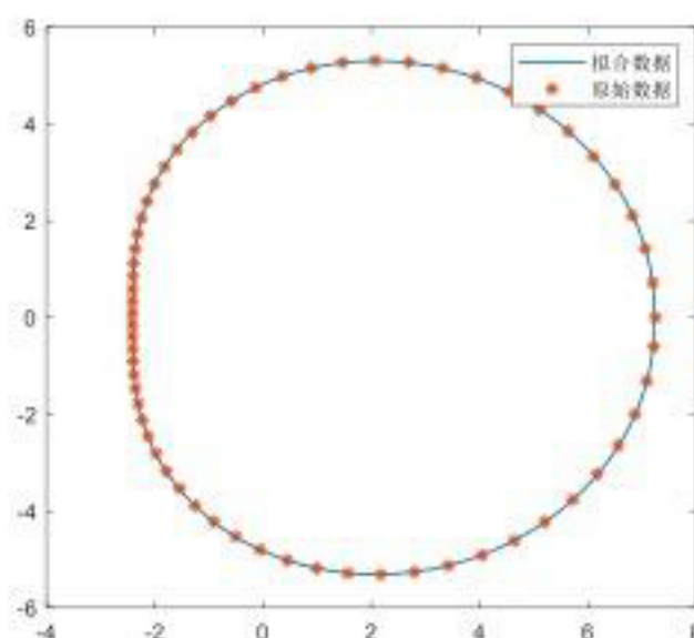
图 10 凸轮边缘曲线图
