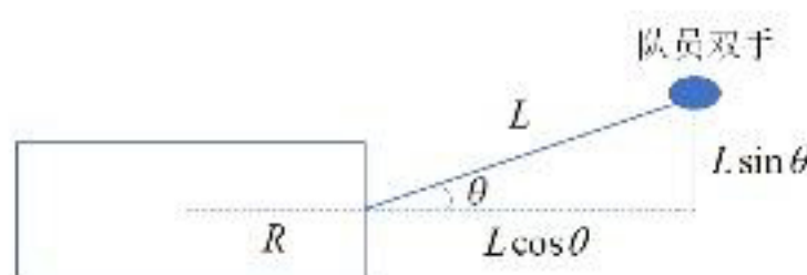
侧视图
