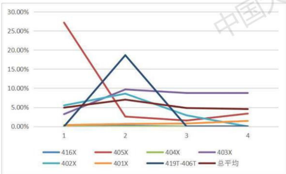
图 14、各子网漏损比率随季度走势图（2σ）
