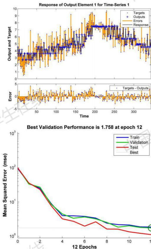
图 19、第五食堂漏损预测
