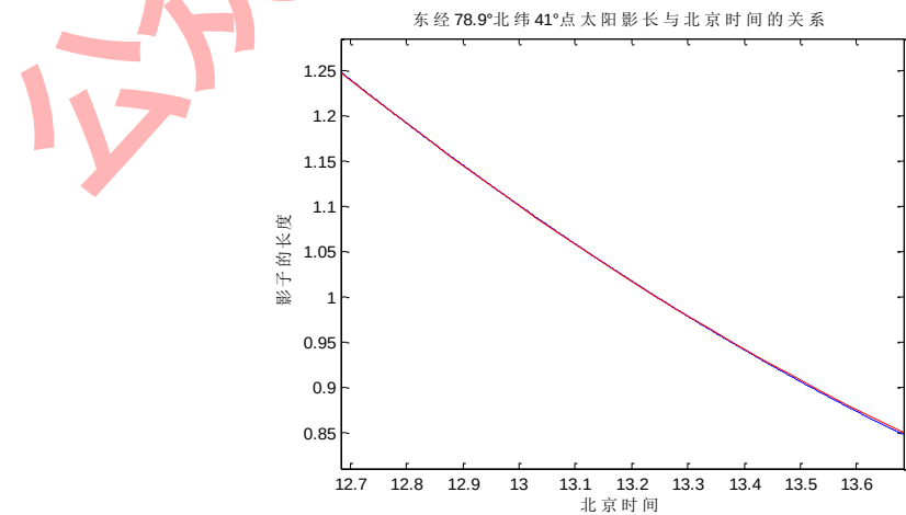
图 14 计算影长与实际影长的对比曲线
