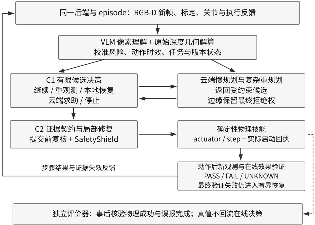
图 1 在线验证驱动的执行决策闭环及独立物理评价
