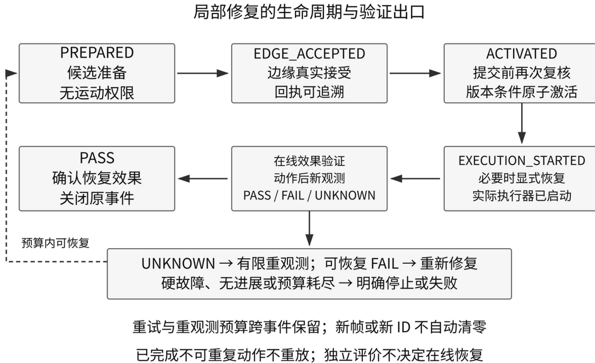
图 2 局部修复的接受 激活 启动与效果验证
