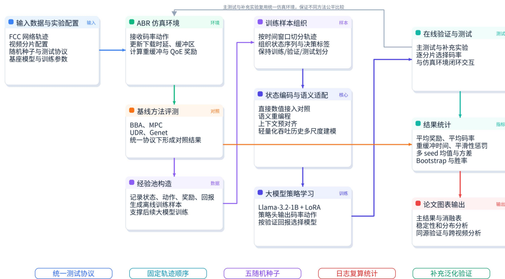
图 2.1 系统架构图
