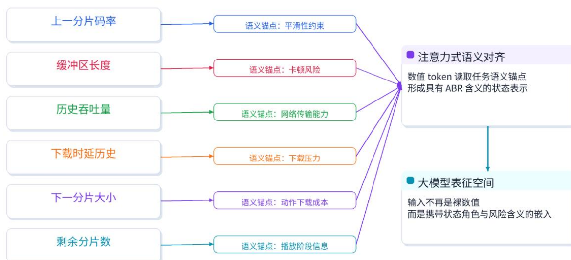
图 3.2 ABR 数值状态的语义重编程映射
