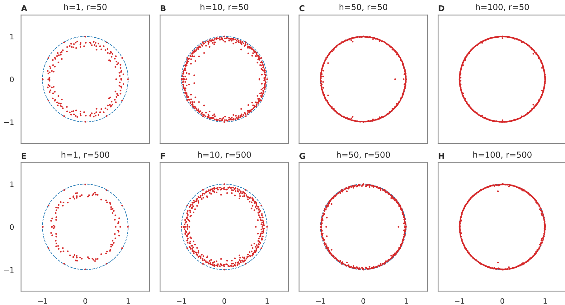
DMD Eigenvalues across Hyperparameters for Hidden Layer 3
