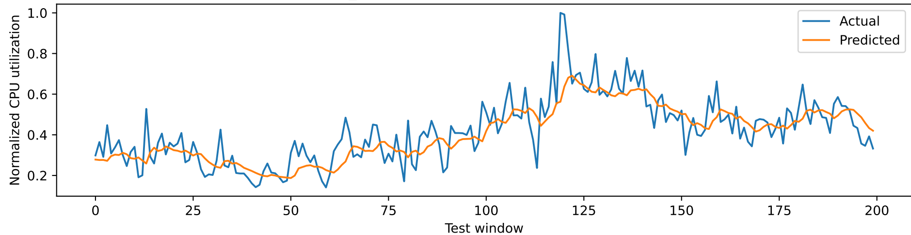
CNN_LSTM: 1-step-ahead forecast vs actual
