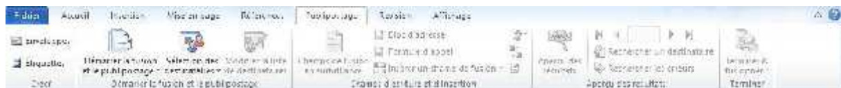
Figure 21 – L'onglet « Publipostage »
