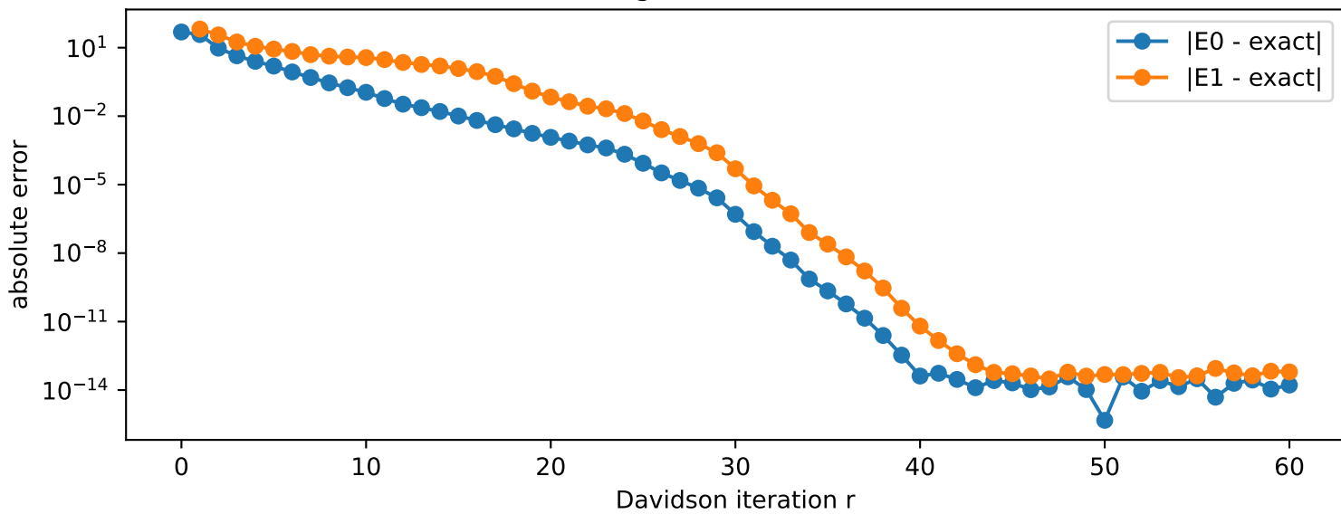
eigenvalue errors
