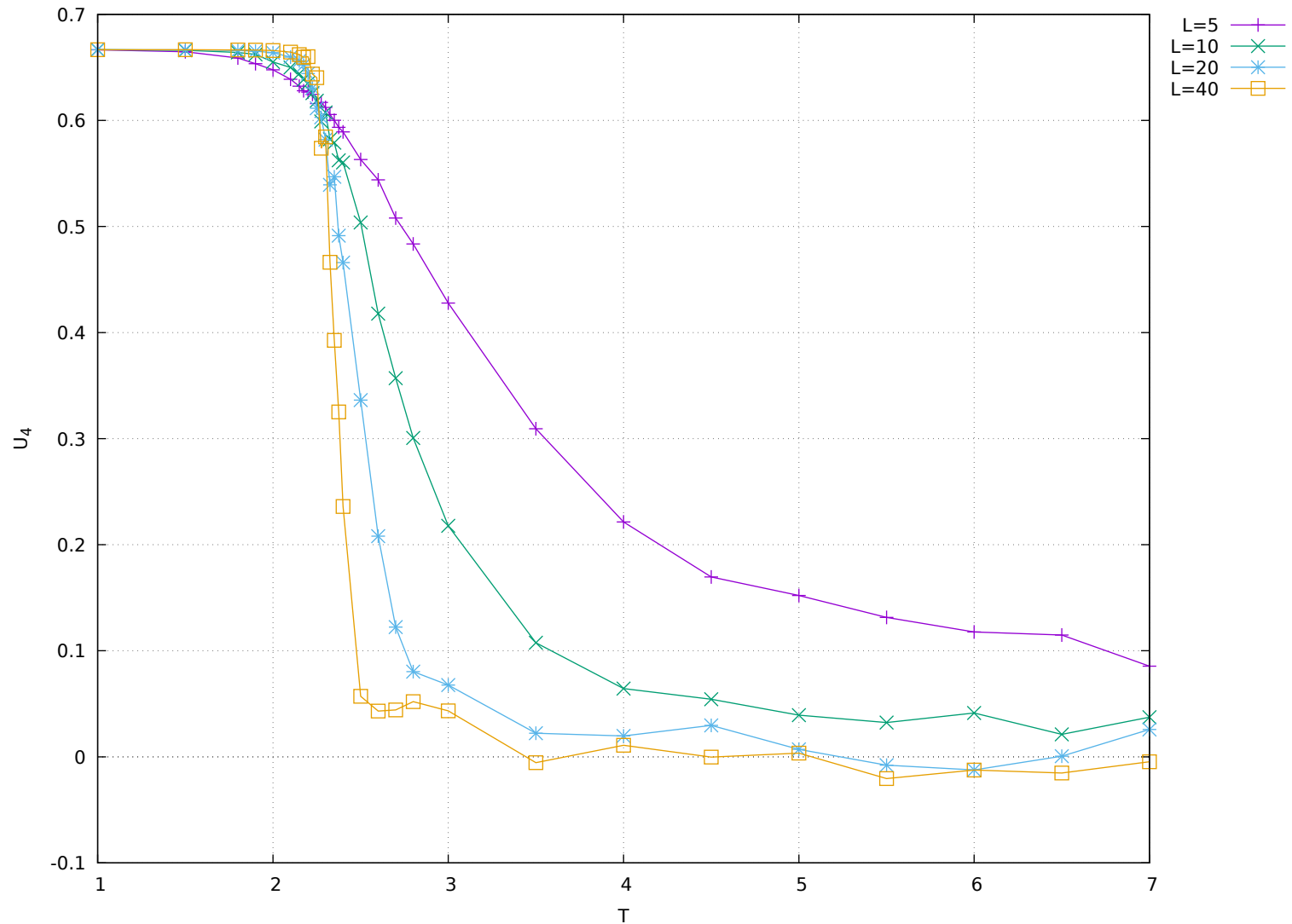
Binder cumulant
