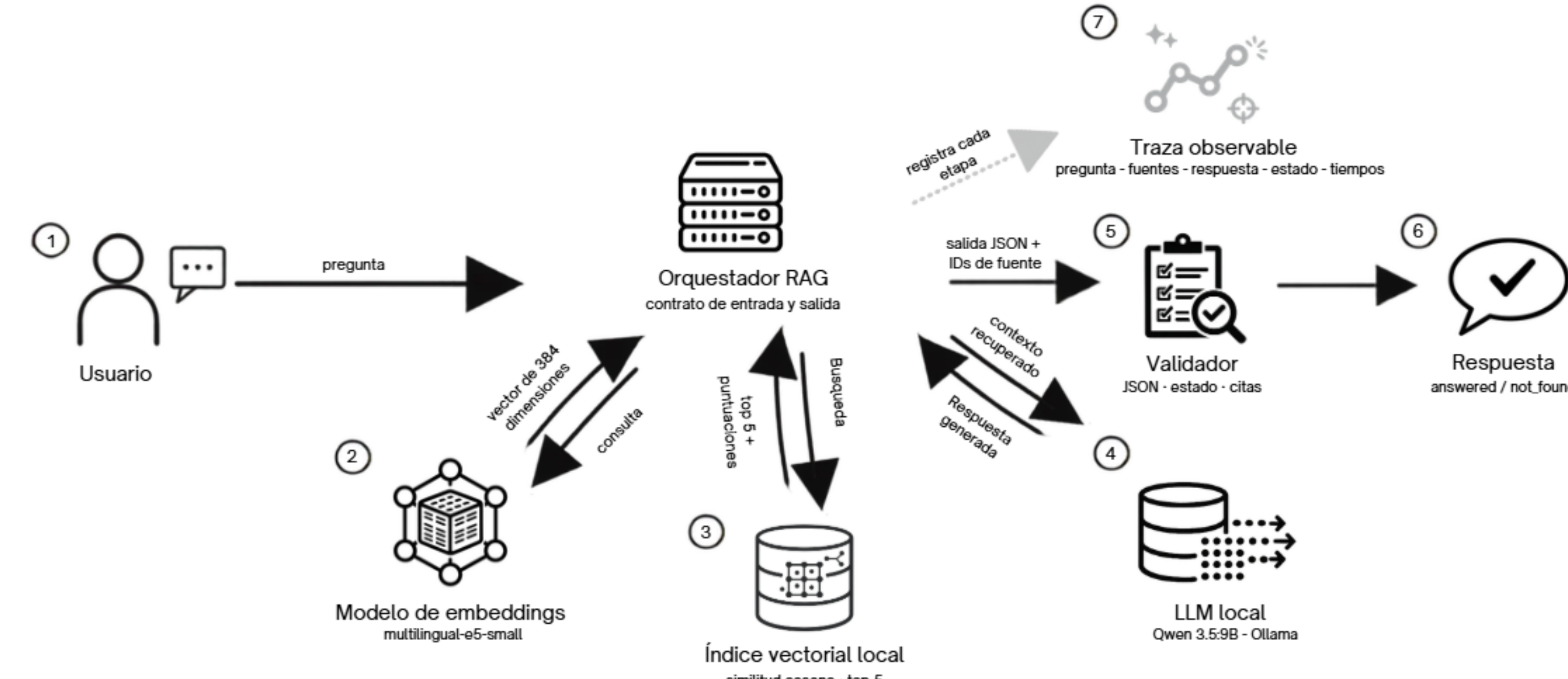
Fig. 2. Flujo observable de consulta y generación. El orquestador coordina la codificación de la pregunta, la recuperación del contexto, la generación local y la validación, mientras conserva los artefactos producidos en cada etapa.
