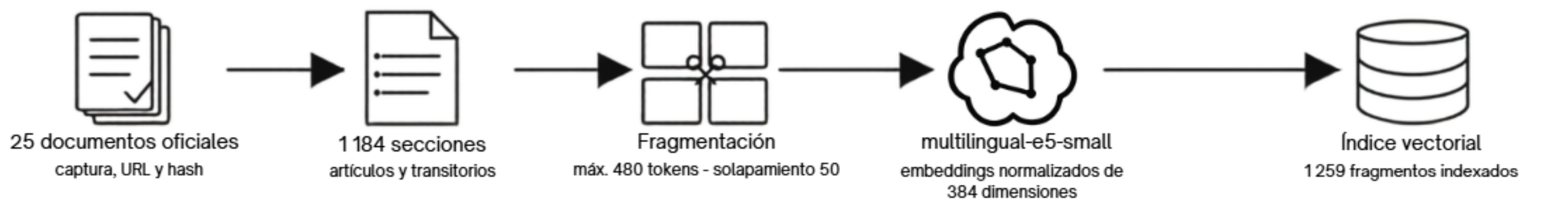
Fig. 1. Indexación reproducible del corpus. Los documentos oficiales se transforman en secciones, fragmentos y representaciones vectoriales normalizadas antes de construir el índice local.
