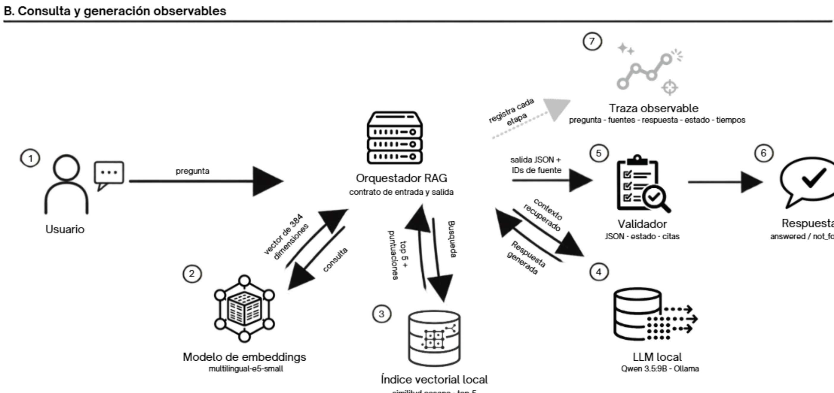
Fig. 2. Flujo de consulta y generación observables. El orquestador coordina embeddings, recuperación, generación y validación; la traza conserva pregunta, fuentes, respuesta, estado y tiempos.
