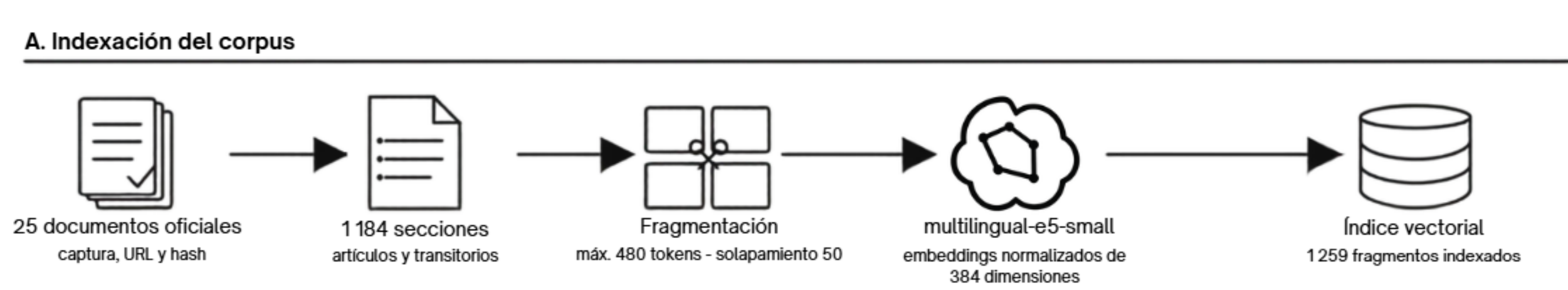
Fig. 1. Flujo de indexación del corpus. Los documentos oficiales se transforman en secciones, fragmentos y embeddings normalizados antes de construir el índice vectorial local.
