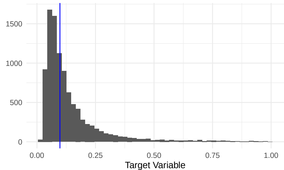
Box-Cox
