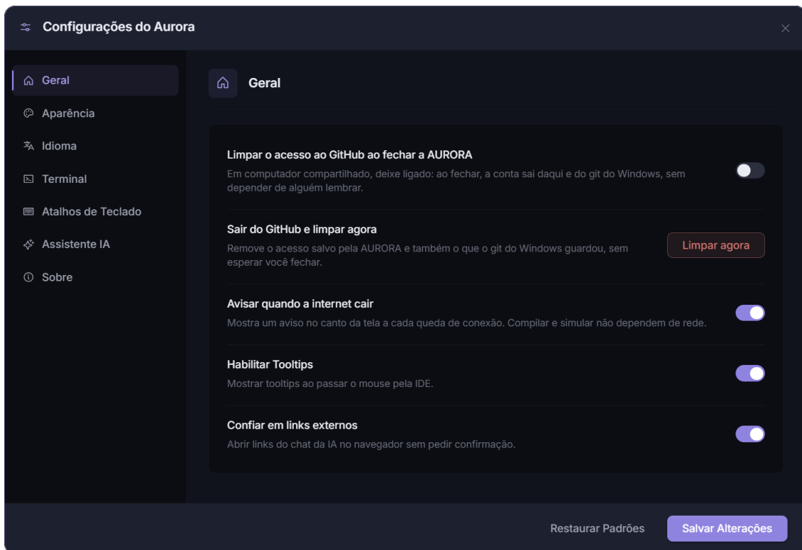
Figura24.1: A aba Geral. As opções de conta do GitHub são as primeiras, porque são as que mais importam em computador compartilhado.
