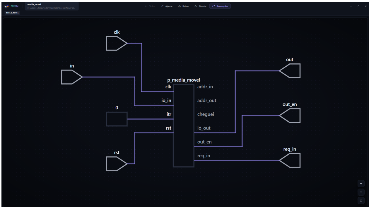
Figura 12.1: O nível do topo. Processadores SAPHO aparecem com símbolo próprio; os demais módulos, como caixas com suas portas.
