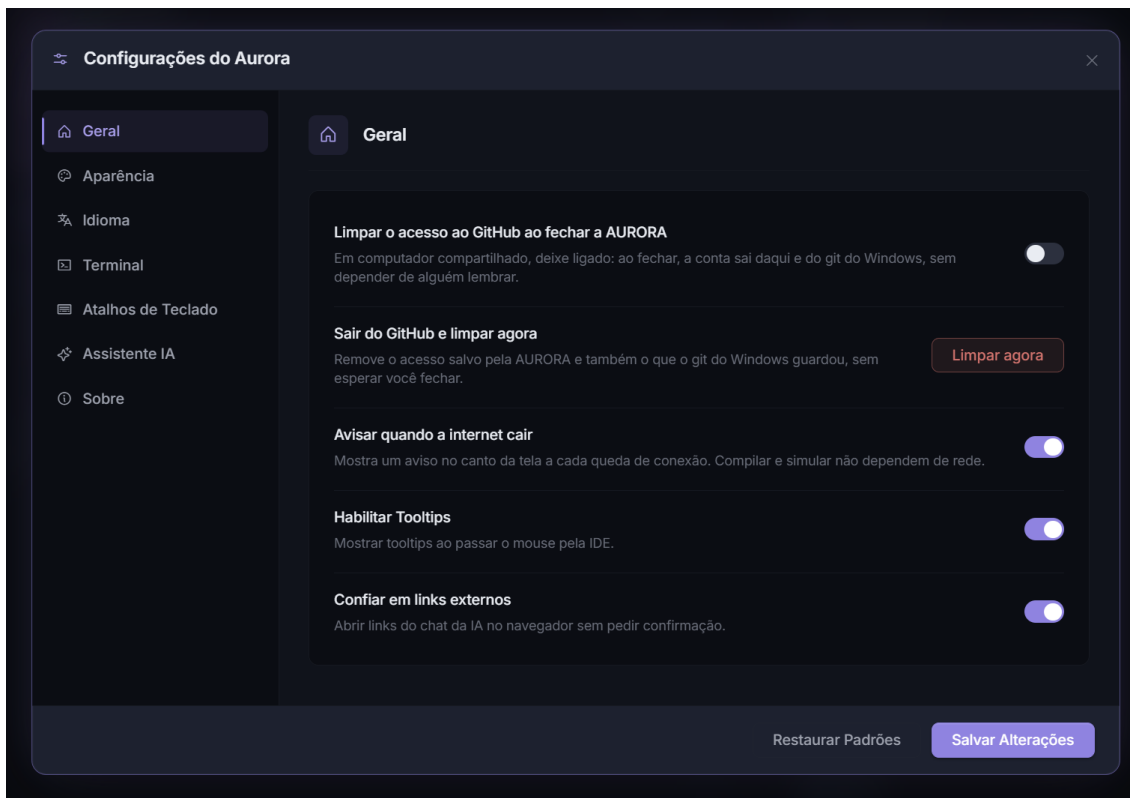
Figura24.1: A aba Geral. As opções de conta do GitHub são as primeiras, porque são as que mais importam em computador compartilhado.
