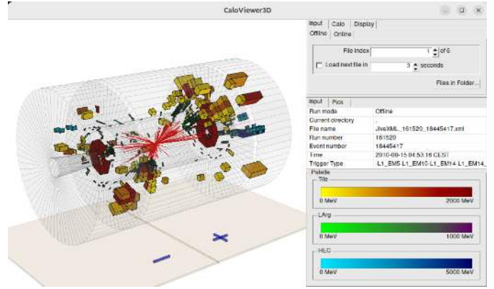
Figura 1. Interface gráfica legada do CGV em ROOT. À esquerda, o visor GL com o calorímetro e as células ativadas pelas partículas incidentens; à direita, o painel de controle.
